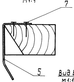
A-A M 1:1
