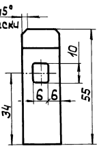
Поз. 5 M1:1
