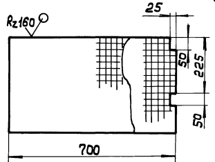
Вид Д
