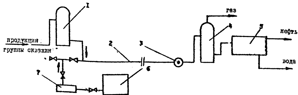
Рис. 5. Схема подачи ингибитора в нефтенпромысловый коллектор. 1-групповая замерная установка; 2-нефтесорный коллектор; 3-пункт контроля; 4-газосепаратор; 5-водоотделитель; 6-ем- кость для ингибитора; 7- дозаторный насос или установка типа БР.
