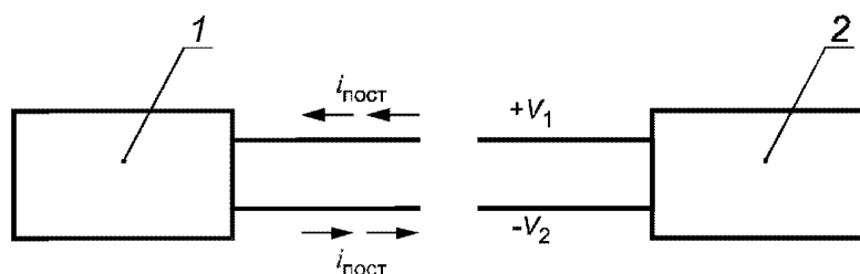
1 — управляющий прибор; 2 — регулируемый ЭПРА
