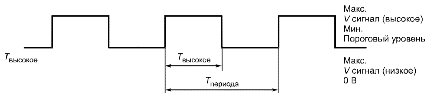
Рисунок Е.5а — Типичный ШИМ-сигнал
