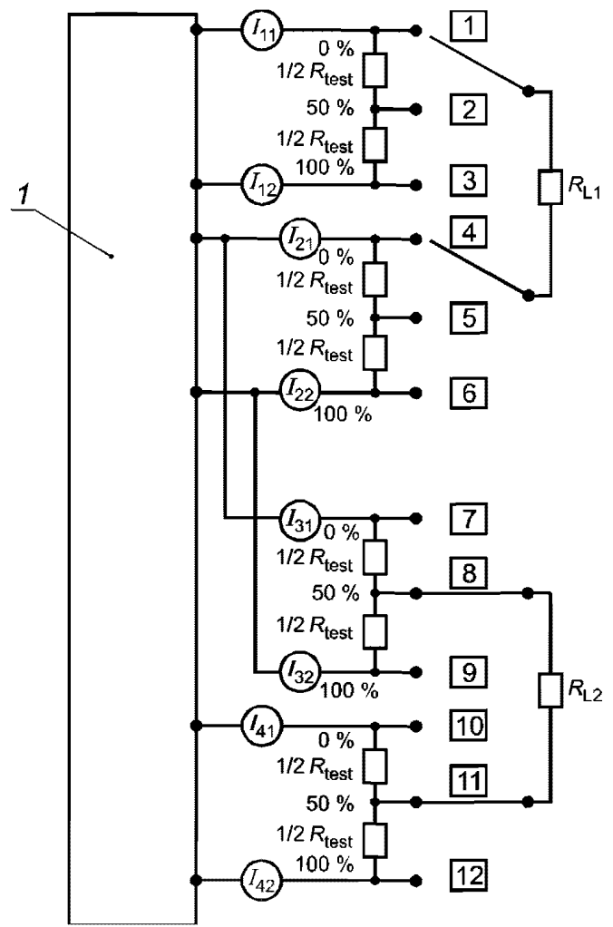
Рисунок F.4b — Электроды, соединенные параллельно
