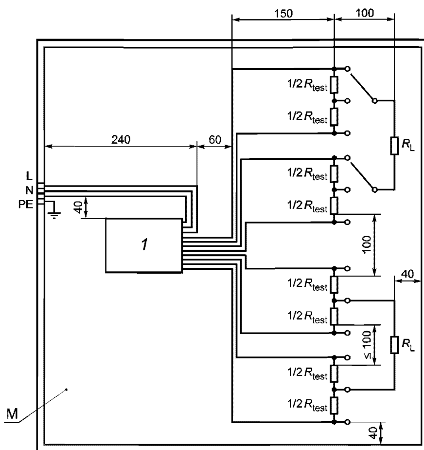
1 — испытуемое устройство (ЭПРА); M — металлическая пластина толщиной 1 мм; R_L — резистор, заменяющий лампу; R_{test} — резистор, заменяющий электрод
