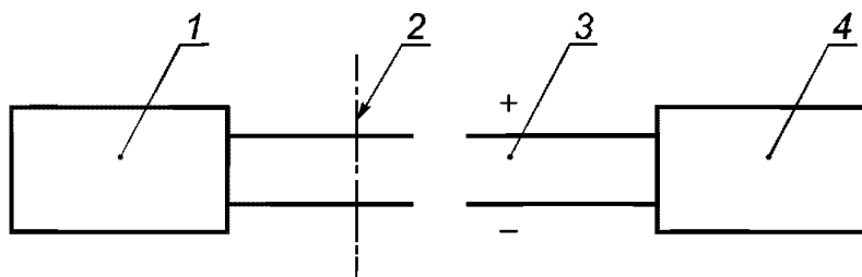
1 — управляющий прибор; 2 — интерфейс; 3 — ШИМ; 4 — регулируемый ЭПРА
