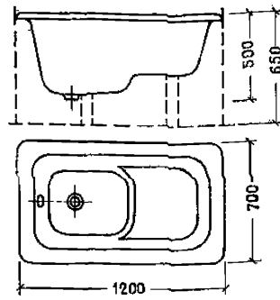
Поддоны: душевые глу- бокие, ГОСТ 10161-62 Тип ПГ
