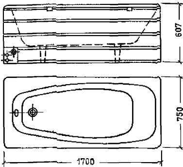
Ванны прямобортные с металличе- ческой панелью, проект ГОСТ а Тип ВН-78
