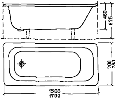
Ванны детские, ГОСТ 1154-66 Тип ДВ-1
