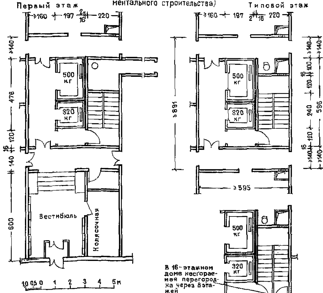
Планировочная схема дома
