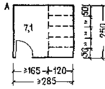
Габаритные схемы помещений для хранения велосипедов, лыж, санок и прочего.
