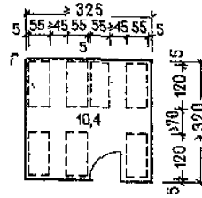
Габаритные схемы помещений для хранения велосипедов, лыж, санок и прочего.
