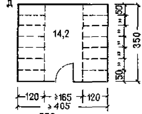
Габаритные схемы помещений для хранения велосипедов, лыж, санок и прочего.
