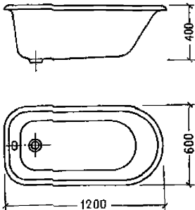
Ванны прямобортные с металличе- ческой панелью, проект ГОСТ а Тип ВН-78
