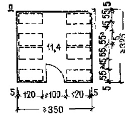
Габаритные схемы колясочных на различное число квартир от 50 до 300 /при средней численности семьи 3,5 чел./
