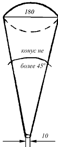
Рис. А.1. Общий вид эклекторной воронки
