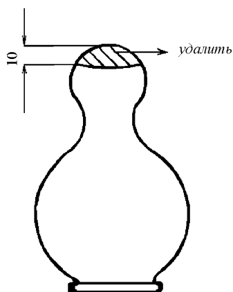
Рис. А.4. Переходник
