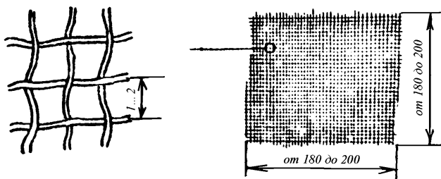
Рис. А.3. Дно электорного сита
