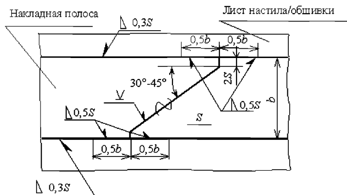
Рис. 5.2.1.3-1 Оформление стыков накладных полос
