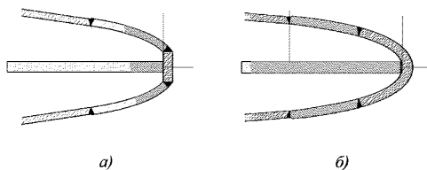
Рис. 3.10.2.6.2-1 Конструкция форштевня: а) комбинированный; б) листовой
