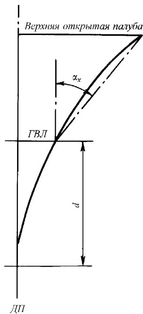
Рис. 2.8.1.2-1 Схема определения угла \alpha_x
