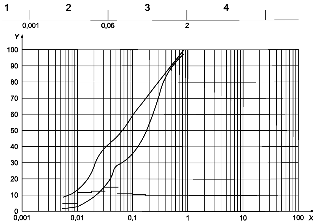
X — диаметр d , мм; Y — пропорция зерен, %, менее d_i ; глина — менее 0,01 мм 2% — 13% по массе; ил — 0,063 мм 30% — 50% по массе; песок — менее 0,25 мм 60% — 78% по массе; гравий — менее 0,5 мм 87% — 90% по массе
