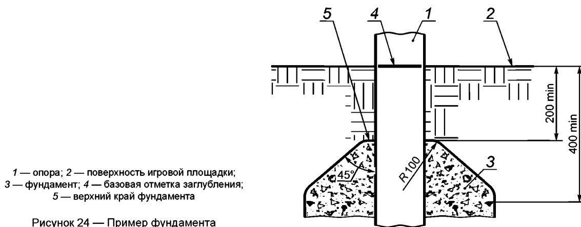
Рисунок 24 — Пример фундамента
