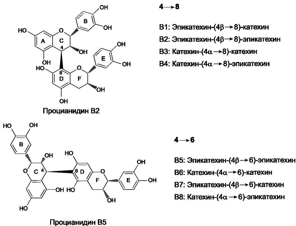
Рисунок А.2 — Структуры проантоцианидинов В-типа
