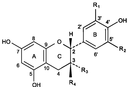
Рисунок А.1 — Структура основных флаван-3-олов
