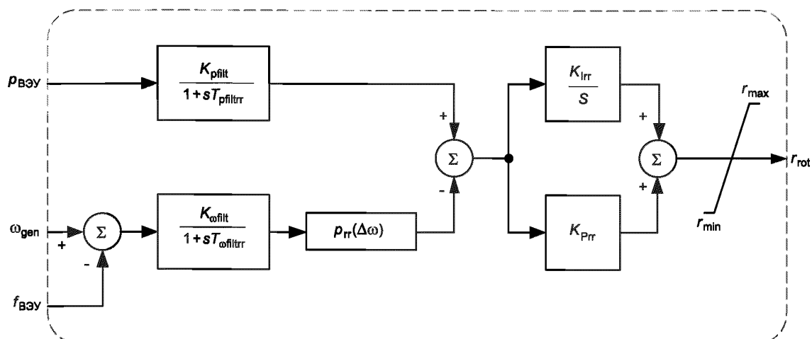
Рисунок 29 — Структурная схема модели регулирования сопротивления ротора генератора
