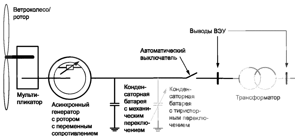
Рисунок 8 — Основные электрические и механические компоненты ВЭУ типа 2
