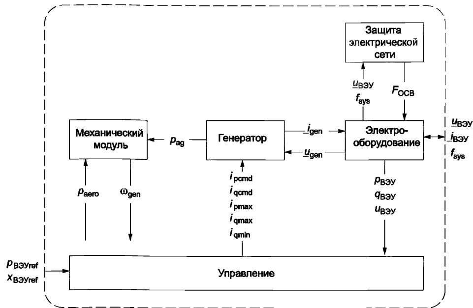
Рисунок 17 — Структура модели ВЭУ типа 4В
