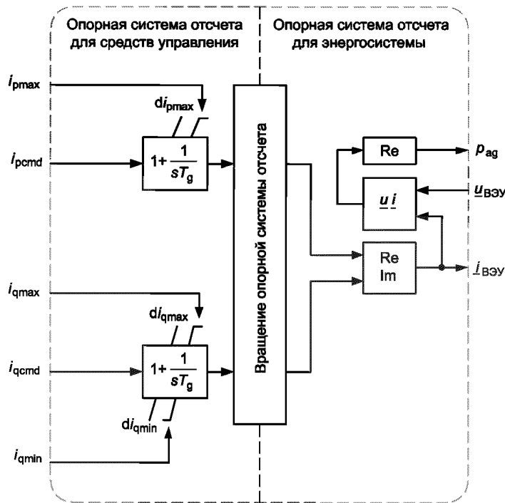
Рисунок 25 — Структурная схема модели генератора ВЭУ типа 4
