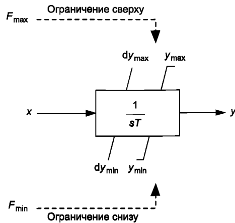
Рисунок В.11 — Обозначение интегратора с ограничениями
