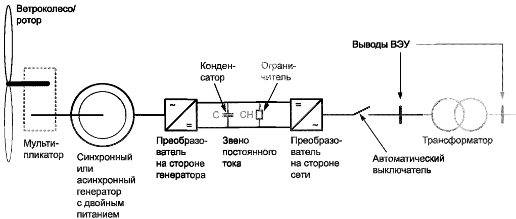
Рисунок 14 — Основные электрические и механические компоненты ВЭУ типа 4
