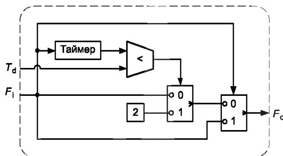
Рисунок В.17 — Структурная схема реализации индикации задержки
