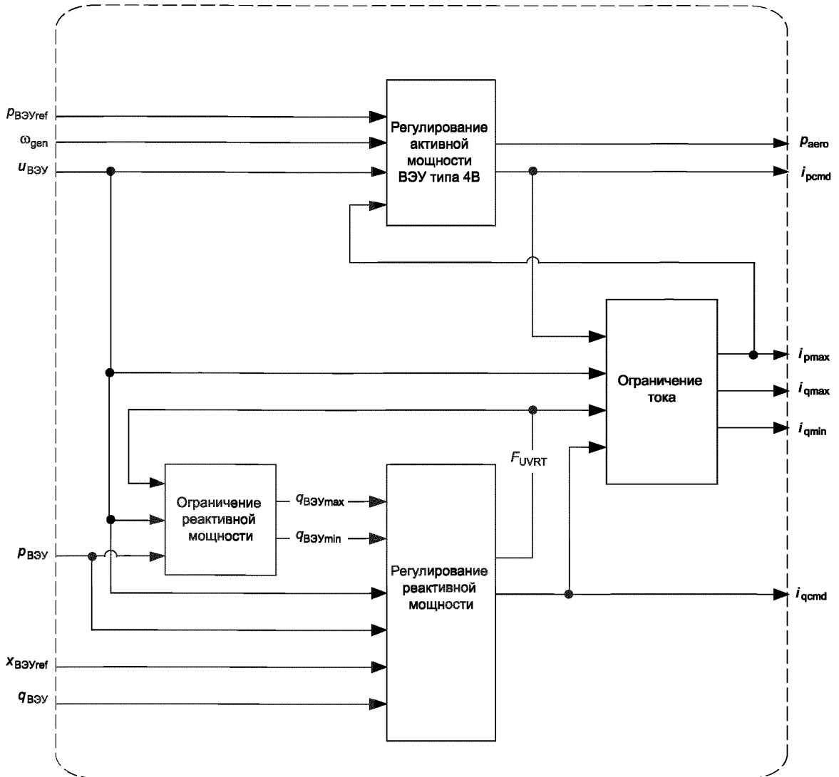
Рисунок 18 — Структурная схема модуля управления модели ВЭУ типа 4В (используется модель ограничения реактивной мощности)
