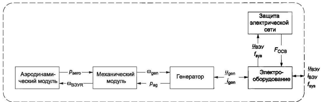
Рисунок 6 — Структура модели ВЭУ типа 1А
