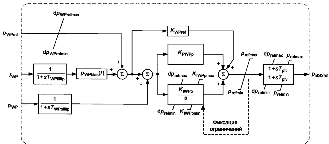
Рисунок А.2 — Структурная схема регулятора активной мощности ВЭС
