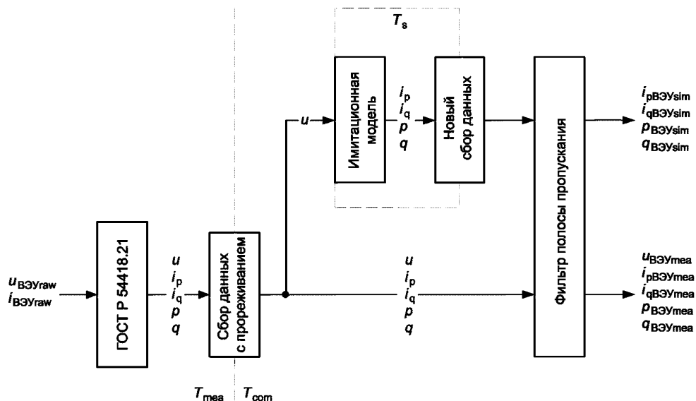
Рисунок 40 — Структура обработки сигналов при применении метода воспроизведения
