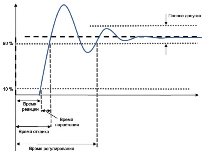
Рисунок 1 — Пример переходного процесса
