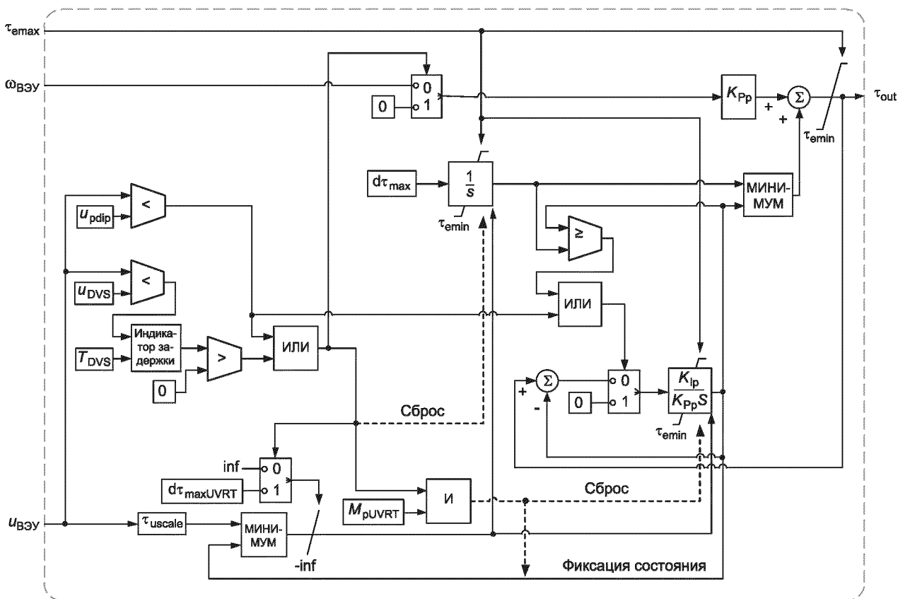
Рисунок 31 — Структурная схема ПИ-регулятора момента
