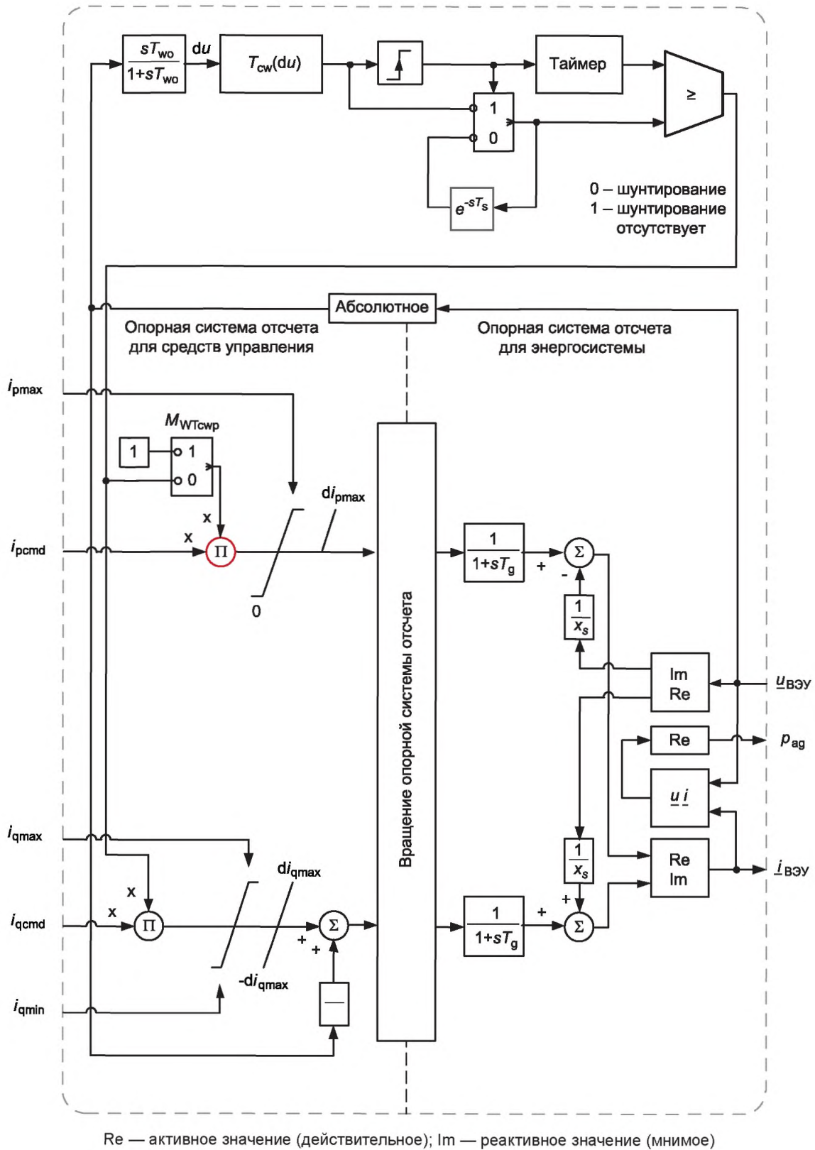
Рисунок 24 — Структурная схема модели генератора ВЭУ типа 3В
