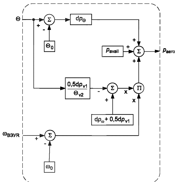
Рисунок 21 — Структурная схема двухпараметрической аэродинамической модели
