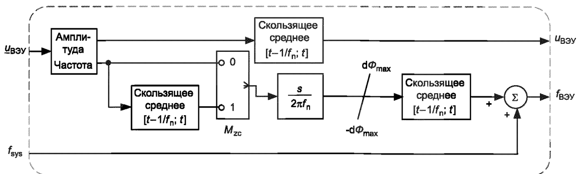
Примечание — Параметр f_n является общим параметром моделей ВЭУ (см. таблицу 1).
