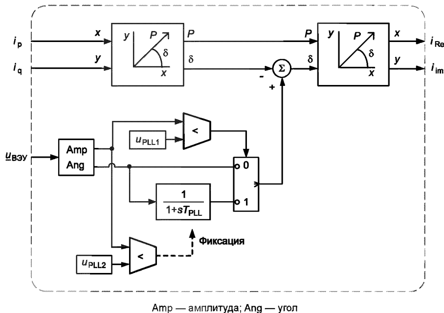
Рисунок 26 — Структурная схема модели вращения опорной системы отсчета
