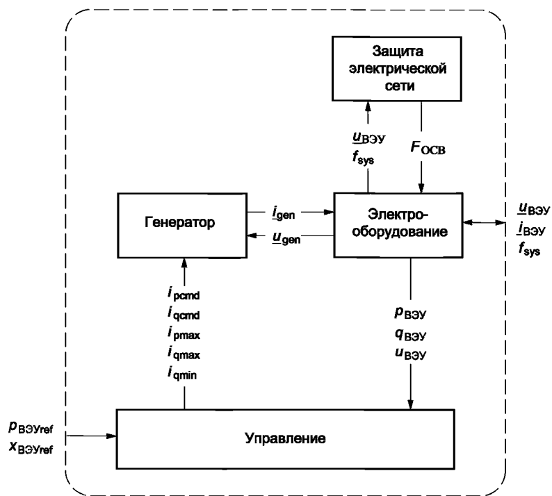
Рисунок 15 — Структура модели ВЭУ типа 4А
