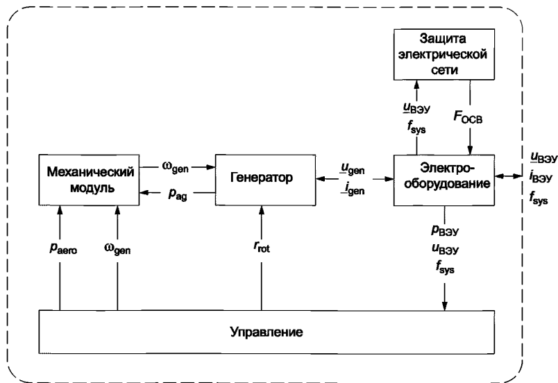
Рисунок 9 — Структура модели ВЭУ типа 2
