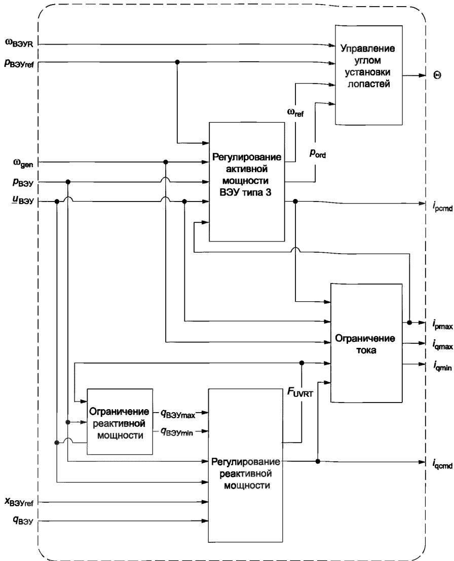
Рисунок 13 — Структурная схема модуля управления моделями ВЭУ типа 3 (используется модель ограничения реактивной мощности)
