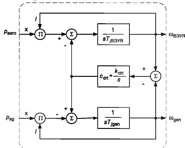
Рисунок 22 — Структурная схема двухмассовой модели
