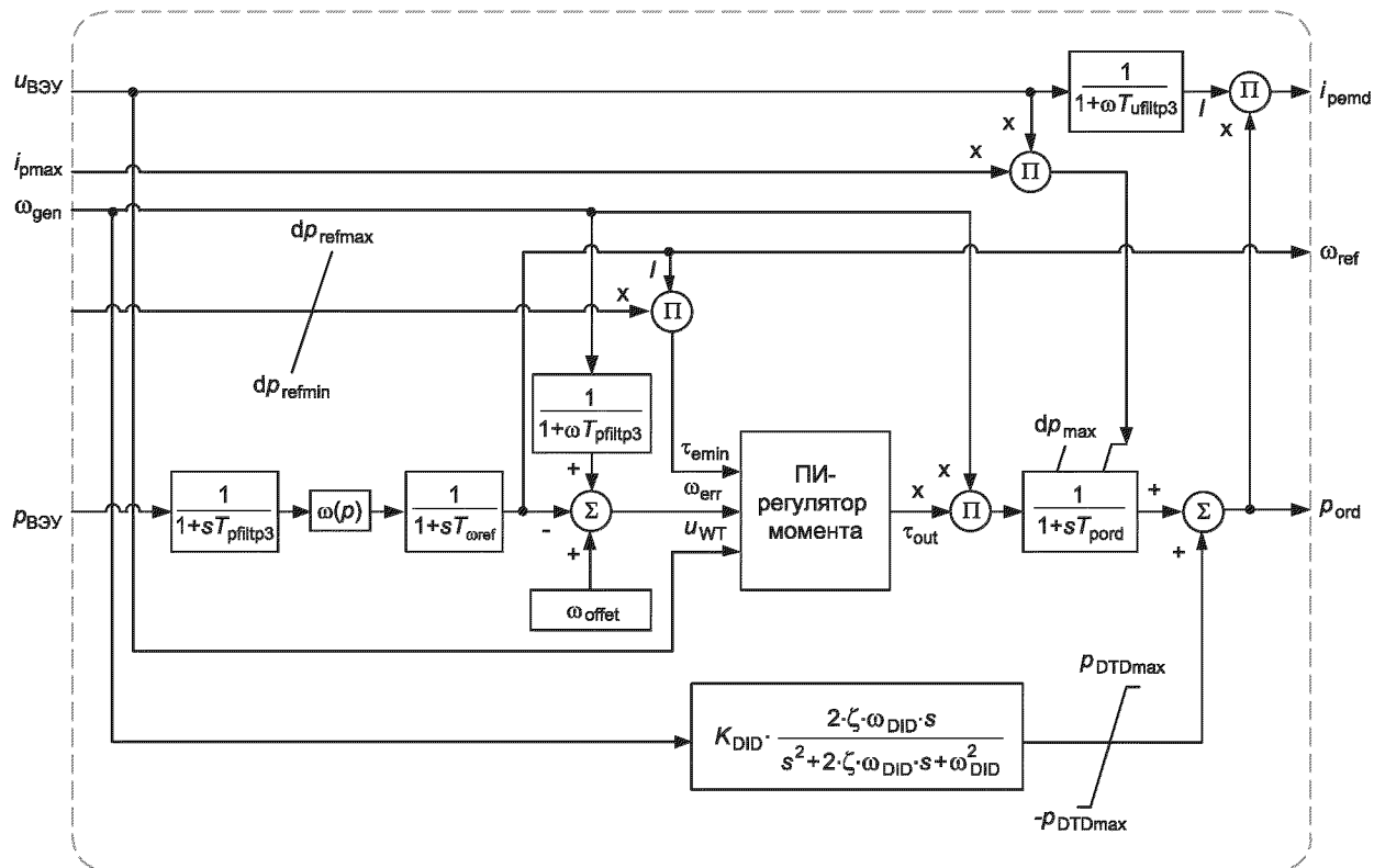
Пр и м е ч а н и е — Звено ПИ-регулятора момента приведено на рисунке 31.
