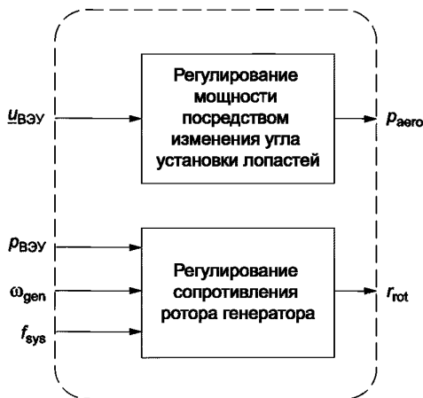
Рисунок 10 — Структурная схема модуля управления модели ВЭУ типа 2
