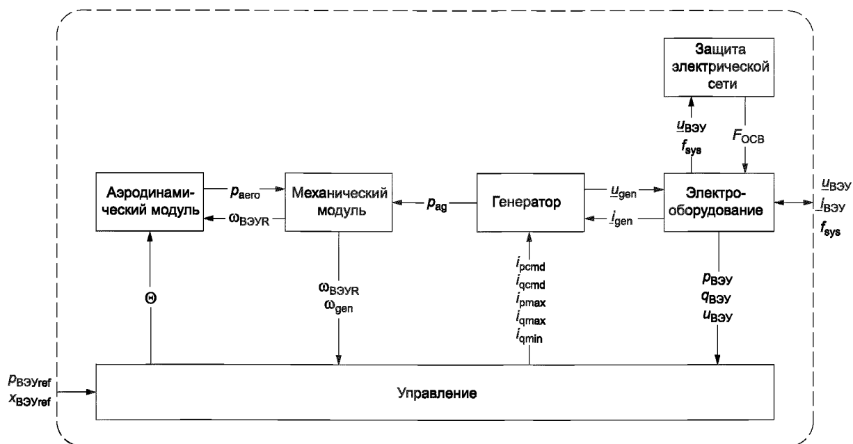
Рисунок 12 — Структура моделей ВЭУ типов 3А и 3В
