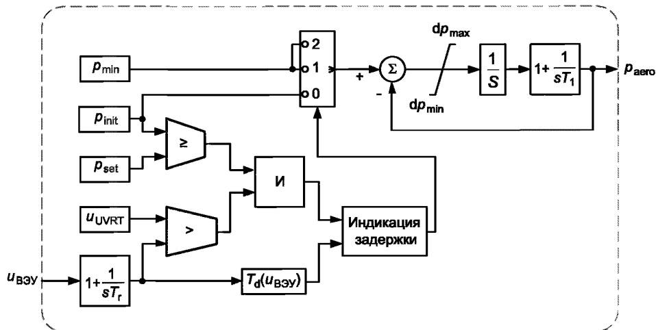
Рисунок 27 — Структурная схема модели управления мощностью углом установки лопастей
