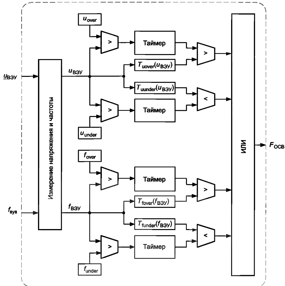
Примечание — Структура звена измерения напряжения и частоты показана на рисунке 39.
