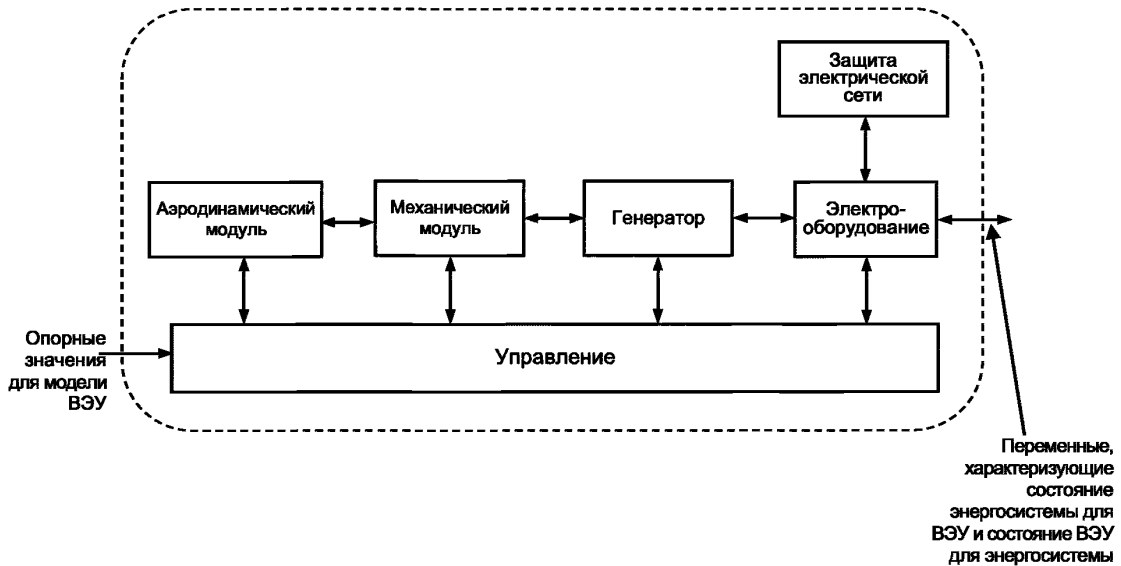
Рисунок 4 — Общая структура моделей ВЭУ
