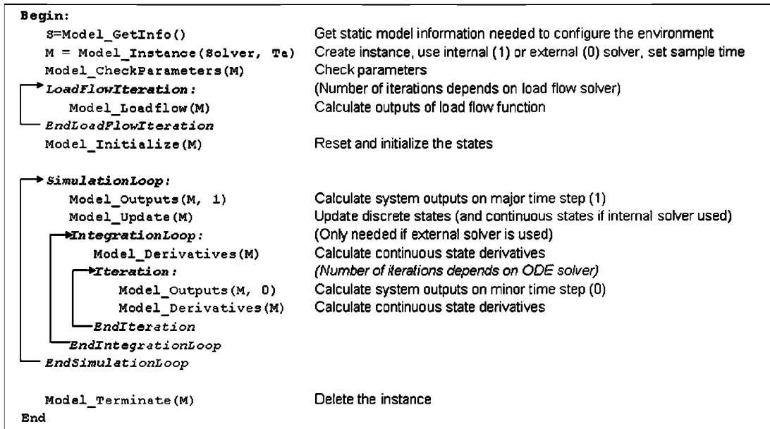
Рисунок G.1 — Последовательность моделирования при использовании PCM-сопряжения
