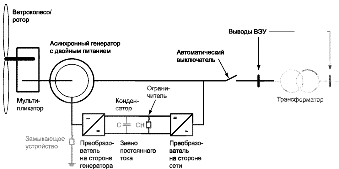
Рисунок 11 — Основные электрические и механические компоненты ВЭУ типа 3
