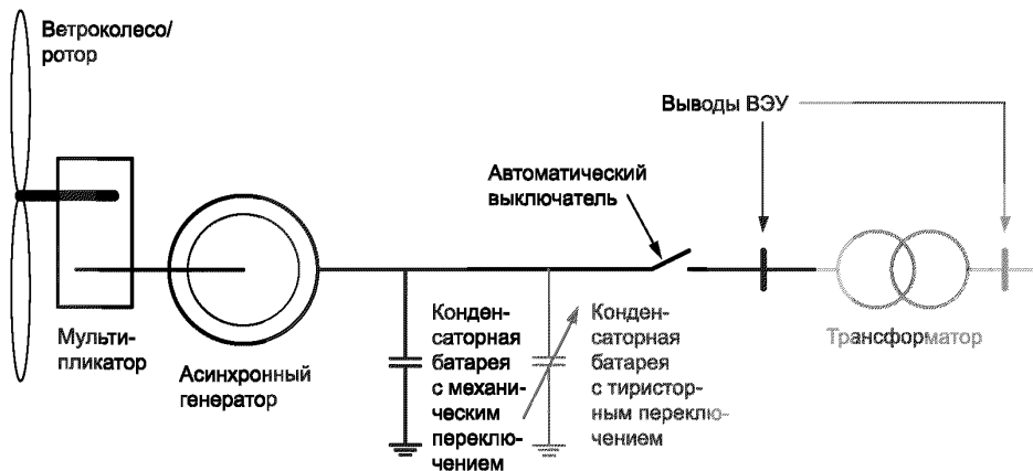
Рисунок 5 — Основные электрические и механические компоненты ВЭУ типа 1
