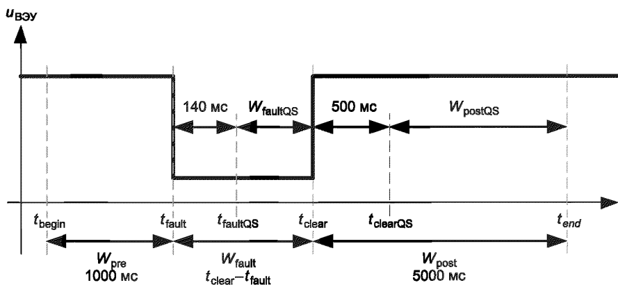
Рисунок 42 — Временные интервалы провала напряжения
