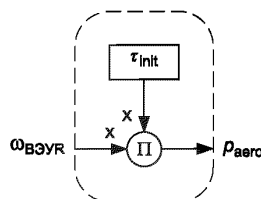
Рисунок 19 — Структурная схема модели с постоянным аэродинамическим моментом
