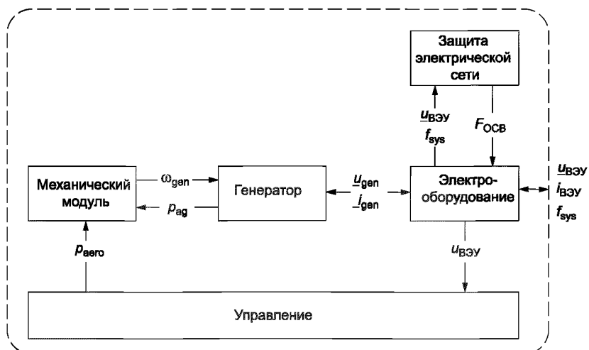
Рисунок 7 — Структура модели ВЭУ типа 1В
