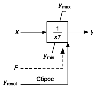
Рисунок В.13 — Обозначение интегратора со сбросом
