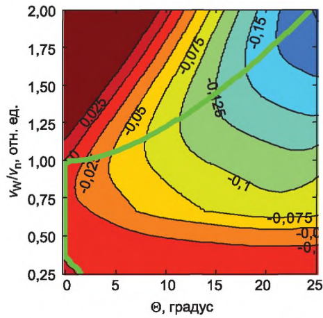
Рисунок С.2 — Зависимость частной производной мощности по угловой скорости вращения ветроколеса/ротора \partial P_{aero} / \partial \omega_R от угла установки лопастей \Theta и скорости ветра v
