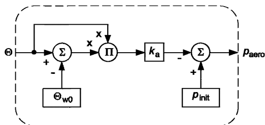
Рисунок 20 — Структурная схема однопараметрической аэродинамической модели
