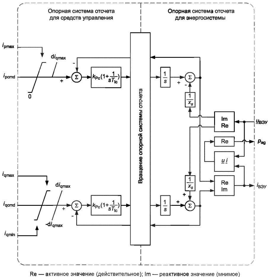
Рисунок 23 — Структурная схема модели генератора ВЭУ типа 3А
