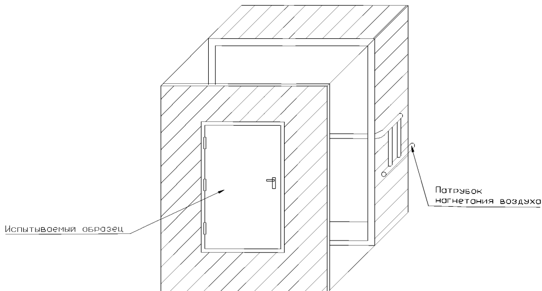
Рисунок А.1 — Схема испытательной камеры
