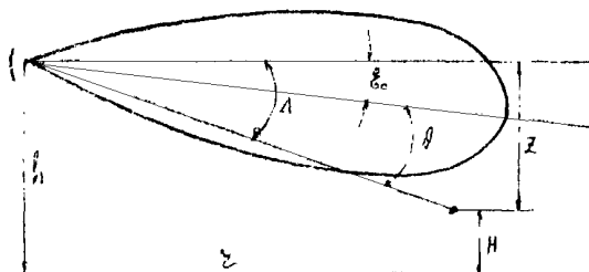
рис. 3.1 Обозначения к расчету ШЭЭЭП.
