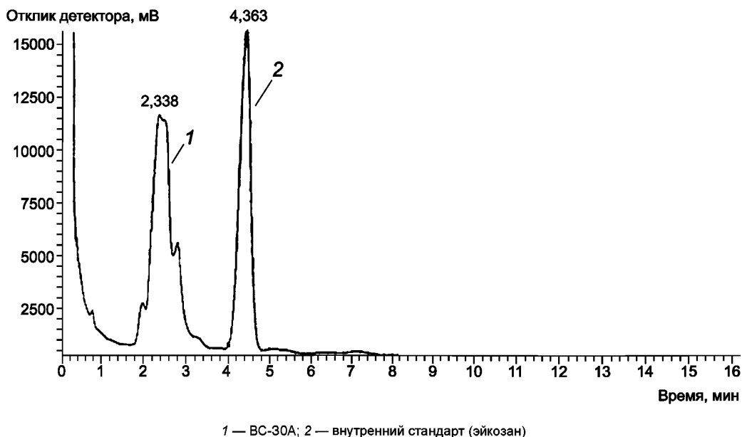
Рисунок 1 — Хроматограмма определения содержания антиоксиданта ВС-30А
