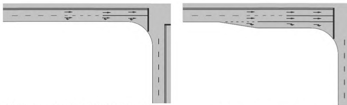
а) Совмещенная полоса прямого движения и правого поворота
