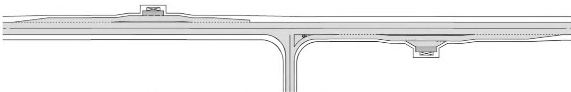
Рисунок 24 — Пример расположения автобусных остановок вблизи примыкания
