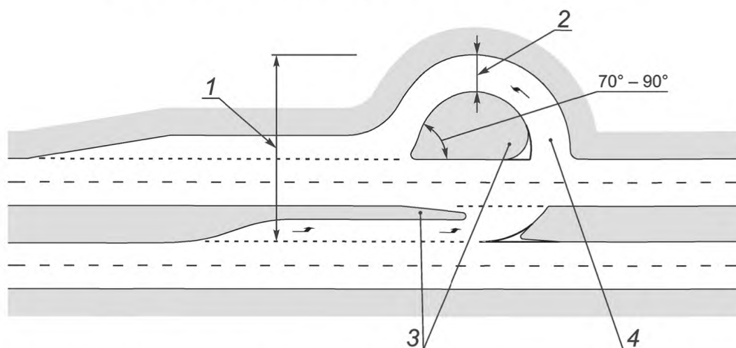
1 — расстояние не менее 32 м для расчетного транспортного средства типа автопоезд А20; 2 — ширина разворота не менее 6,5 м для грузовых транспортных средств; 3 — геометрия островка и центральной разделительной полосы, определяемая по габаритам поворачивающих транспортных средств; 4 — геометрия разворота, определяемая по габаритам поворачивающих транспортных средств при скорости движения 5—15 км/ч
