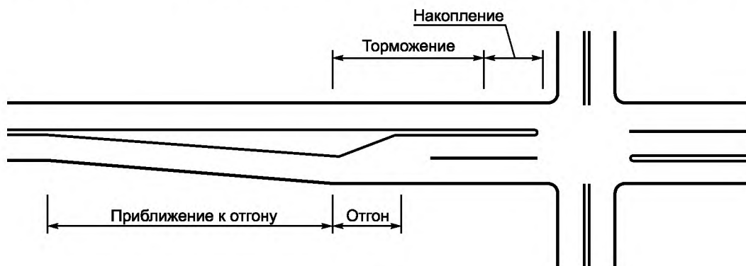
Рисунок 9 — Полоса для поворота налево при наличии центральной разделительной полосы
