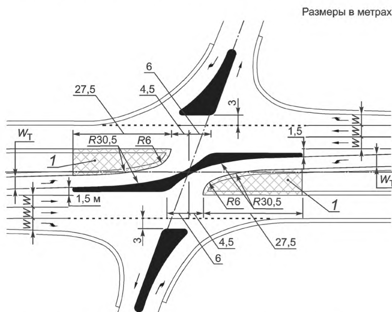
Рисунок 19 — Пересечение в одном уровне с отнесенными левыми поворотами с второстепенной дороги и левым поворотом с главной дороги без обеспечения прямого проезда по второстепенному направлению
