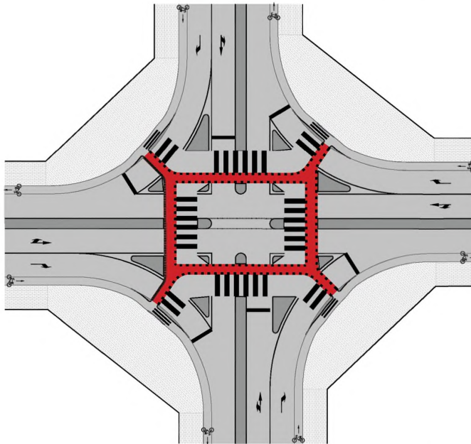
Рисунок 21 — Совмещение пешеходных путей и велосипедных дорожек
