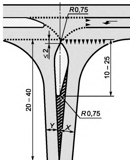
Рисунок 14 — Схема построения центрального направляющего островка, используемого как с целью направления движения, так и с целью безопасного движения пешеходов
