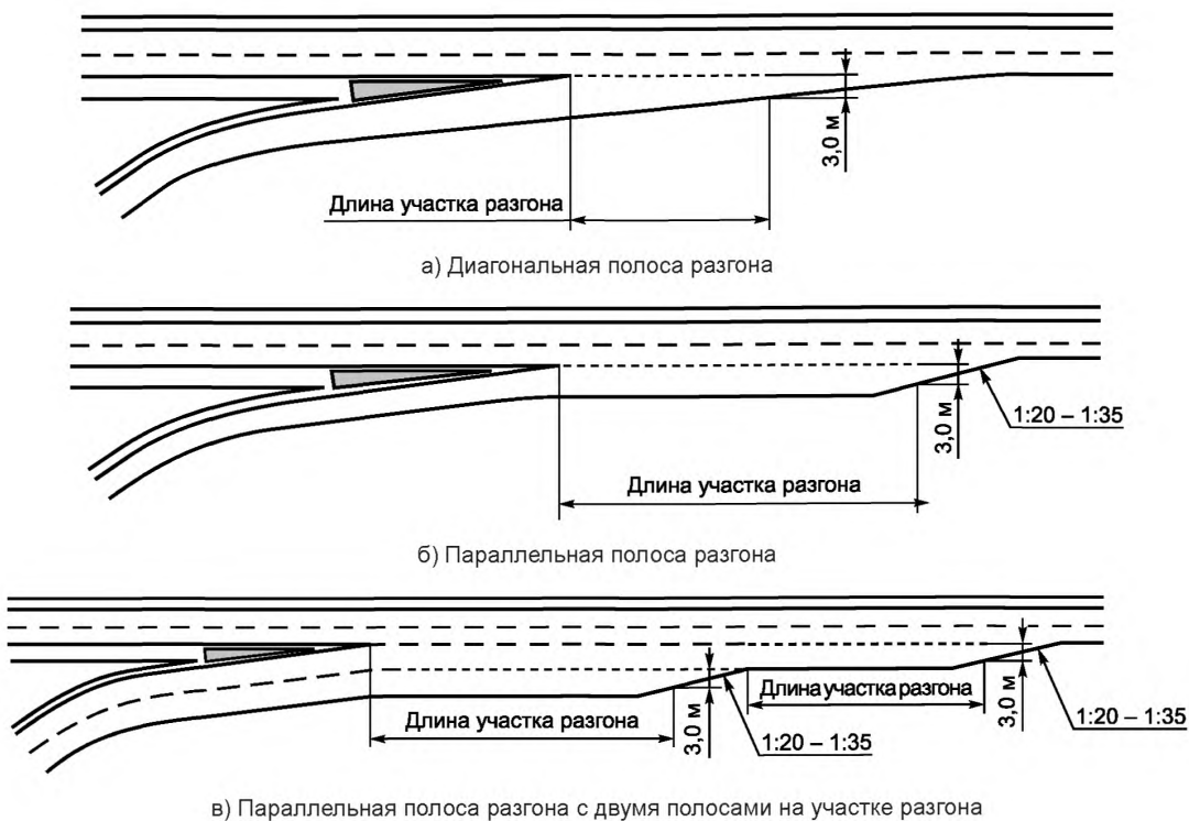
Рисунок 7 — Схема организации полосы разгона для поворота направо
