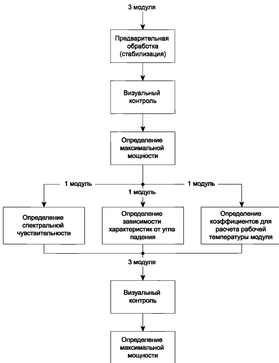
Рисунок 1 — Порядок проведения испытаний (параллельное выполнение основных испытаний)
