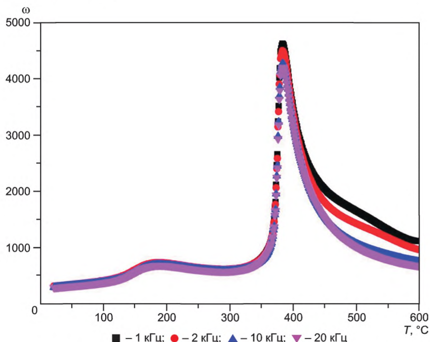
Рисунок А.2 — Зависимости \epsilon'/\epsilon_0(T) и \epsilon''/\epsilon_0(T) в частотном интервале f = (1 \div 20) кГц
