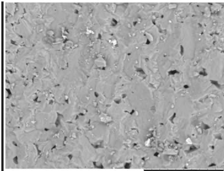
Рисунок А.1 — Микротография зеренной структуры керамики NKCNO-1. Маркер — 30 мкм
