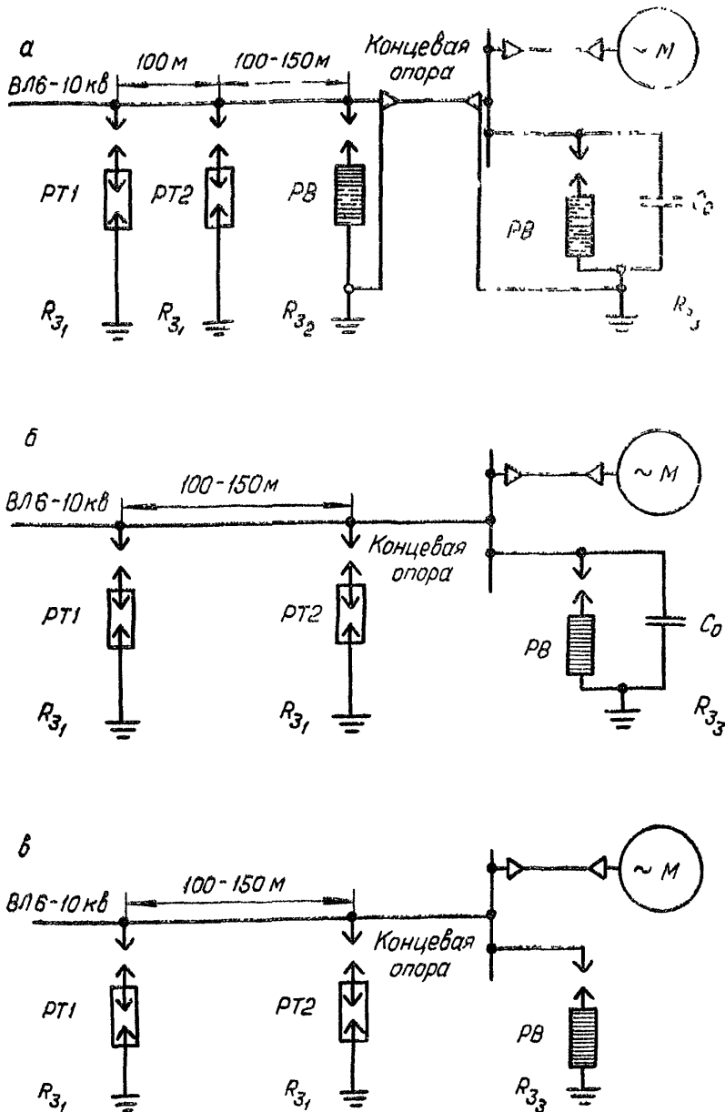
Рис. 6. 2 Схемы защиты вращающихся электрических машин, присоединенных к ВЛ 6—10 кВ непосредственно или через короткие (до 50 м) кабельные вставки. R_{з1} — R_{з2} — сопротивление заземления трубчатых и вентильных разрядников; R_{з3} — сопротивление заземления вентильных разрядников (не более 4 Ом); C_0 — защитная емкость (0,5 мкФ/фазу).
