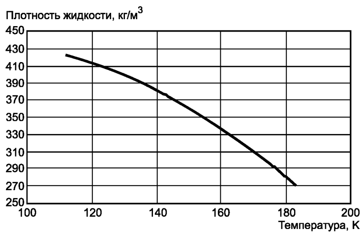
Рисунок А.2 — Плотность жидкого метана
