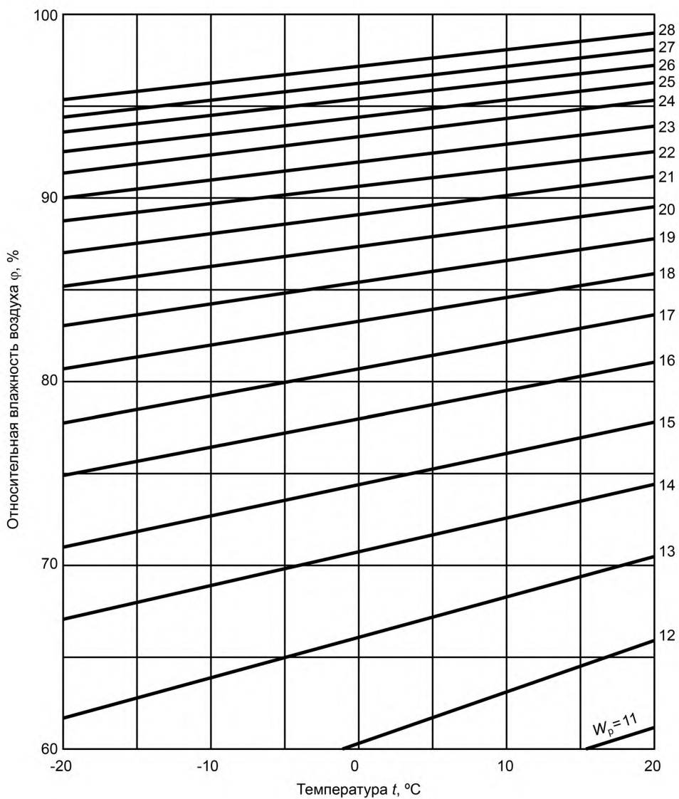
Диаграмма равновесной влажности древесины
