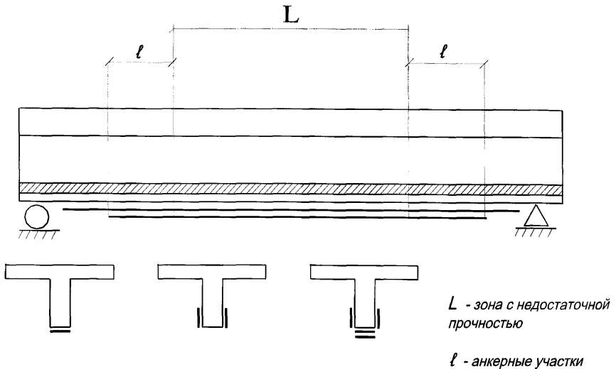
Рис. 2 Схемы усиления, вызванные недостаточной прочностью нормальных сечений
