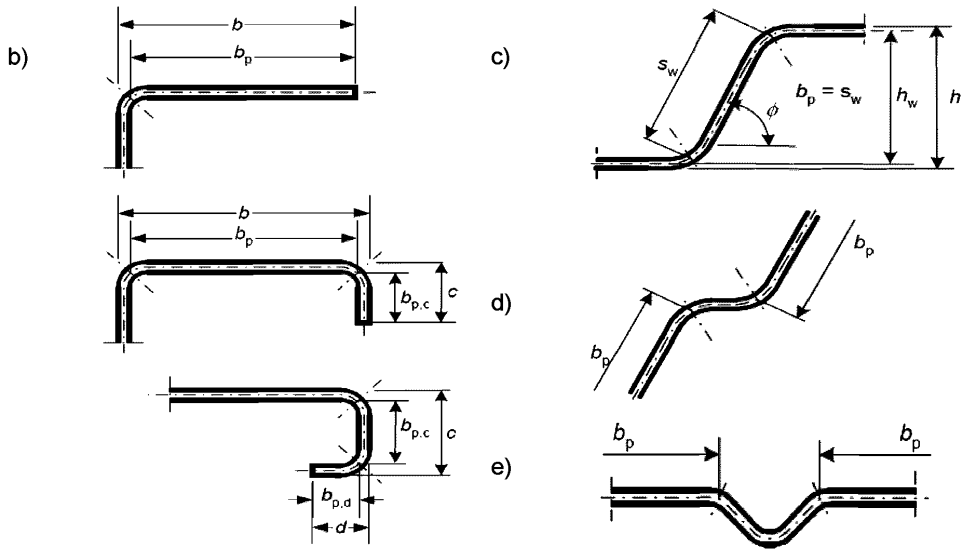
а – средняя точка угла или сгиба; б – теоретическая ширина b_p для плоских частей полок; с – теоретическая ширина b_p плоской части стенки ( b_p = наклонная высота s_w ); д – теоретическая ширина b_p плоских частей, смежных с элементом жесткости на стенке Рисунок 7. 3 – Теоретическая ширина b_p плоских участков поперечного сечения, примыкающих к углу профиля.
