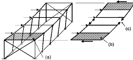
а – настил; б – зона сдвига в настиле; с – усилия в поясах крайних элементов
