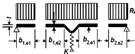
Рисунок В.8 – Схема к этапу I. Эффективные ширины полки при \sigma_{\text{com}} = R_y
