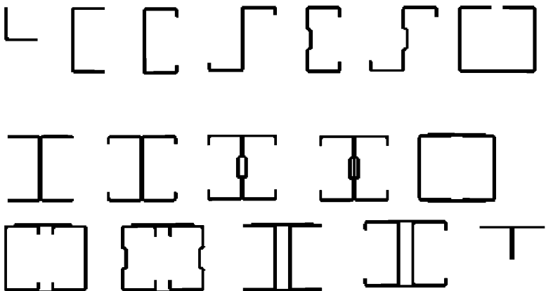
Рисунок 5.1 – Распространенные формы несущих профилей и составных сечений элементов конструкций из стальных тонкостенных холодногнутого профилей
