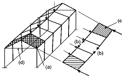
(а) – настил; (б) – усилия в поясах крайних элементов; (с) – зона сдвига в настиле; (д) – затяжка, требуемая для восприятия усилий от кровельного покрытия
