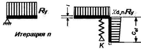
Рисунок В.5 – Схема к этапу III
