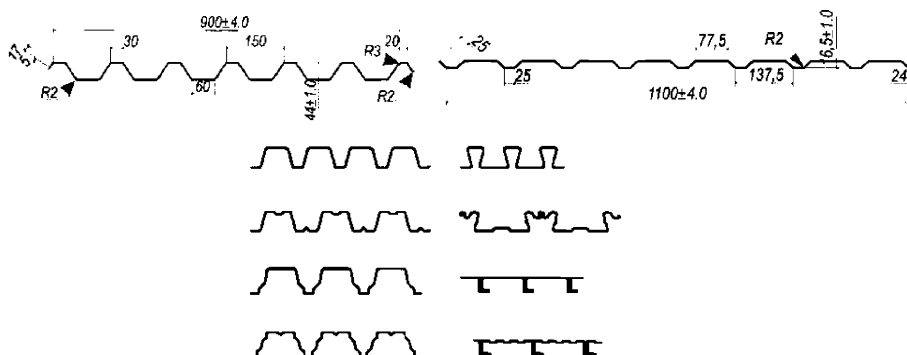
Рисунок 5.2 – Формы сечений профилированных листов и кассетных профилей
