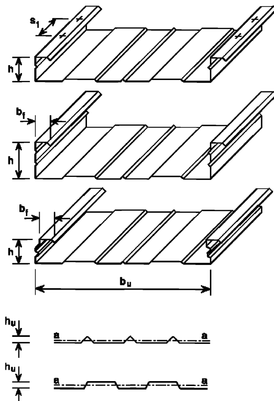
Рисунок 8.1 – Типичная геометрия кассетных профилей
