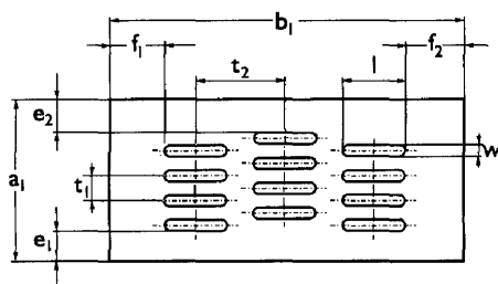
Рис. 10 Lgvl Перфорация с продолговатыми отверстиями в рядах, смещёнными друг относительно друга
