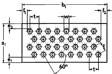
Рис. 2 Rv Круглая перфорация со смещенными рядами отверстий
