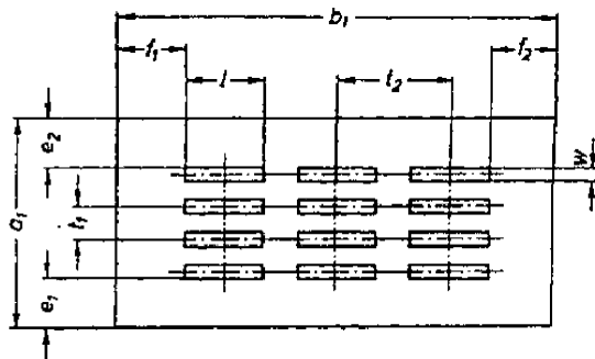
Рис. 7 Lge Прямоугольная перфорация с прямыми рядами отверстий
