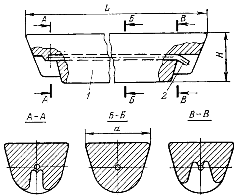
Рис. 1. Конструкция магневых анодов типа ПМ. 1 — анод магневый; 2 — сердечник контактный.
