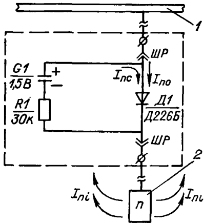
Рис. 7. Схема протекторного вентиля устройства со смещенным порогом открывания 0,3 В. 1 — защищаемое сооружение; 2 — протектор.
