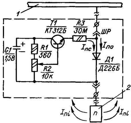
Рис. 8. Схема протекторного вентиля устройства с регулируемым порогом открывания. 1 — защищаемое сооружение; 2 — протектор.
