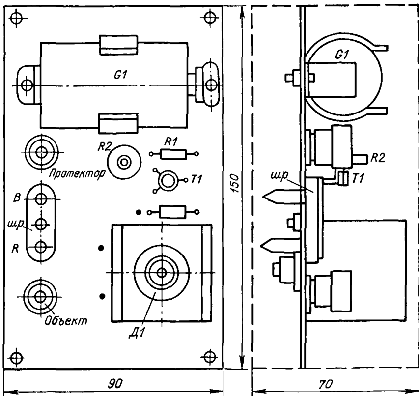
Рис. 9. Общий вид компоновки монтажной платы смещенного вентиля устройства в закрытой коробке.
