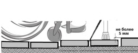
Рисунок 5.3 – Требования к покрытию пешеходных путей движения
