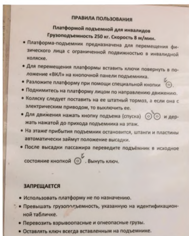
Рисунок 6.91 – Правила пользования платформой и пульт управления платформой
