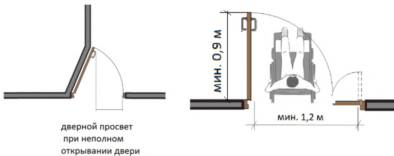
Рисунок 6.50 – Ширина дверного проема и рабочей створки двупольных дверей
