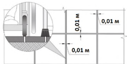
Рисунок 5.3 – Требования к покрытию пешеходных путей движения
