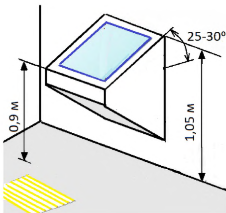
Рисунок 10.26 – Высота размещения тактильной схемы
