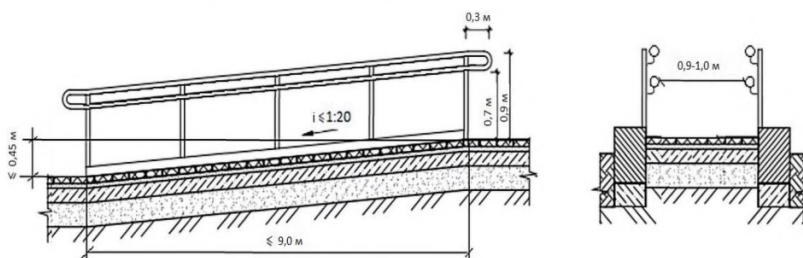
Рисунок 5.19 – Габариты пандуса на рельефе
