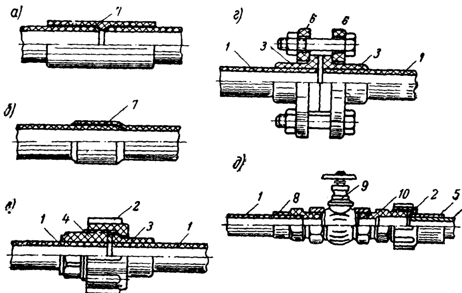
Рис. 3. Соединения винипластовых труб
