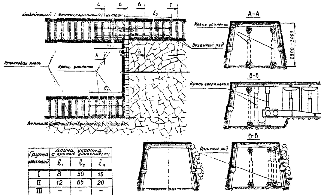
Рис. 14. Паспорт крепления, охраны и поддержания выемочных выработок по второму варианту с трапециевидной крепью ТИЖ.
