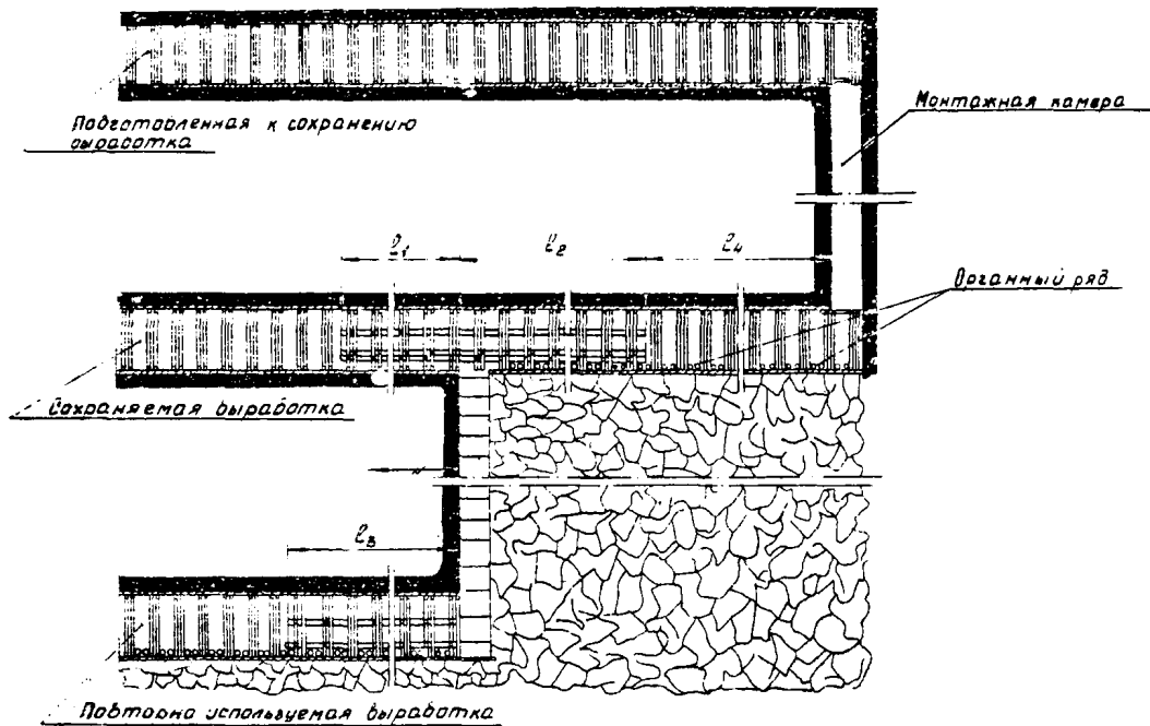
Рис. 10. Схема расположения и крепления выработок, сохраняемых за собой для их повторного использования.
