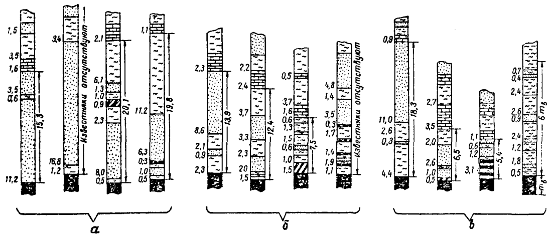
Рис. I. Строение и литологический состав кровли (примеры): легкой (а), средней (б), тяжелой (в)
