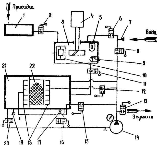
Рис. 4. Гидравлическая схема установки ВНИИНП:
