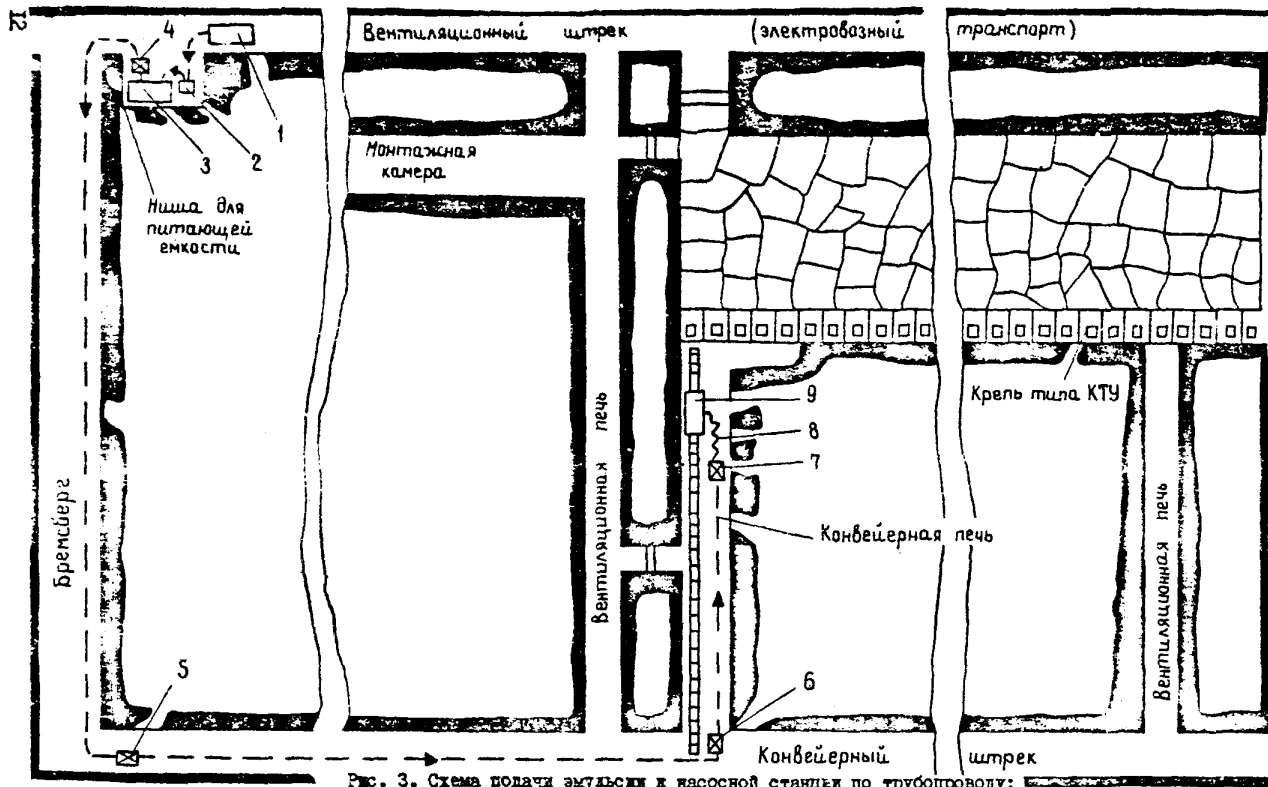
Рис. 3. Схема подачи эмульсии к насосной станции по трубопроводу: 1 - транспортная емкость; 2 - перекачивающее устройство; 3 - питающий бак; 4 - главный ventиль; 5, 6, 7 - магистральные ventильи; 8 - подводный вентиль; 9 - насосная станция
