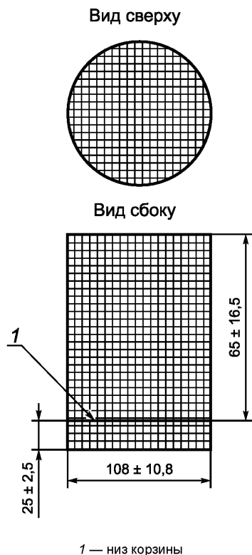
Рисунок 1 — Проволочная корзина
