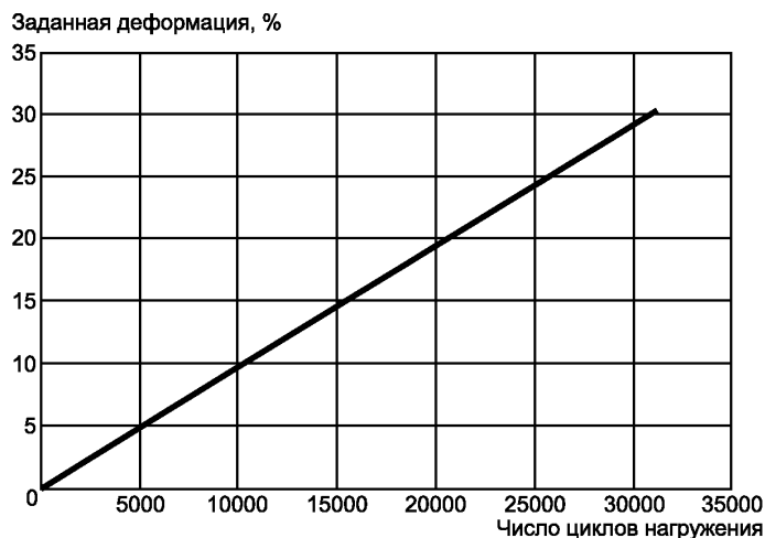
Рисунок 2 — Условия изменения заданной деформации при проведении испытаний
