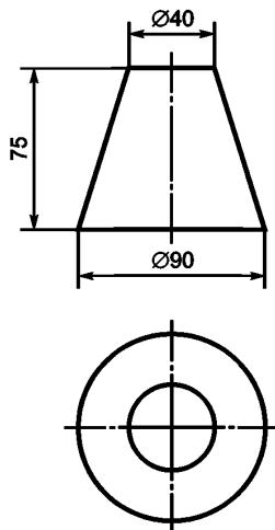
Рисунок 1 — Металлическая форма
