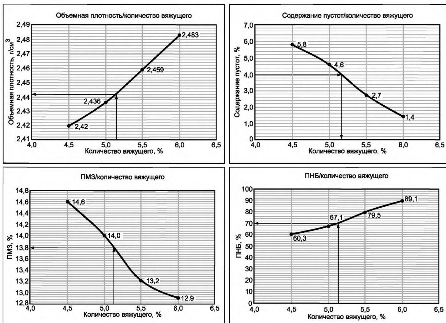
Рисунок Г.1 — Пример построения графиков для выбора оптимального количества вяжущего
