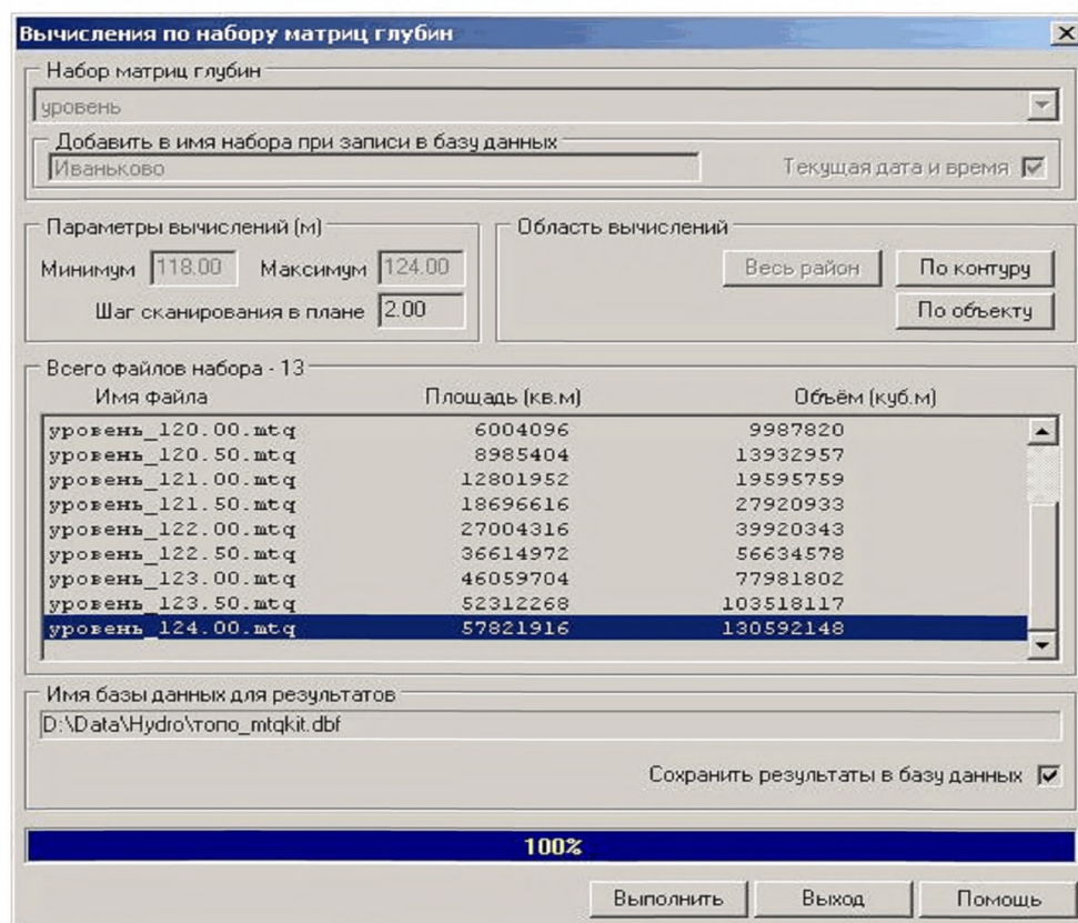
Рисунок 9.9 – Диалоговое окно вычислений по набору матриц глубин
