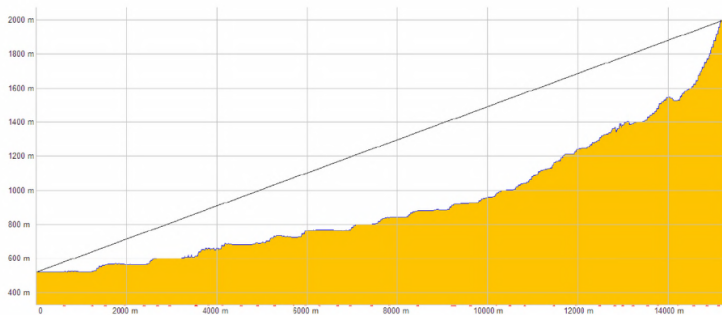
Рисунок В.4 – Продольный профиль реки Вердыз'ерк
