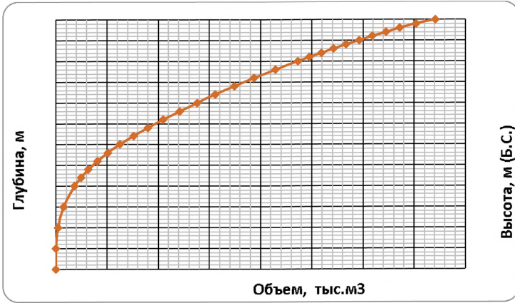
Рисунок 7.8 – Объемная кривая озера Богатырское
