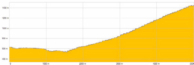
Рисунок В.5 – Поперечный профиль реки Вердыз'ерк в 1,2 км от устья
