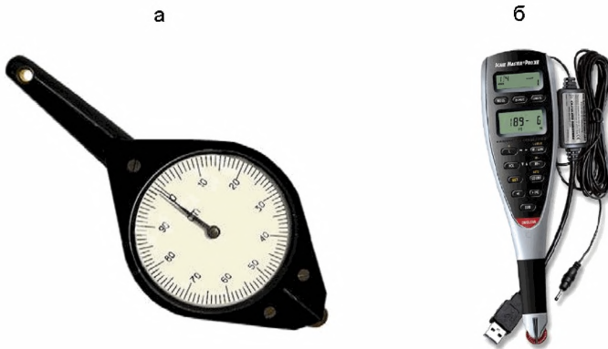
а – курвиметр механический КУ-А;
