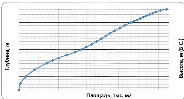
Рисунок 7.7 – Батиграфическая кривая озера Богатырское
