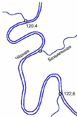
Рисунок 8.3 – Пример определения высоты уреза воды
