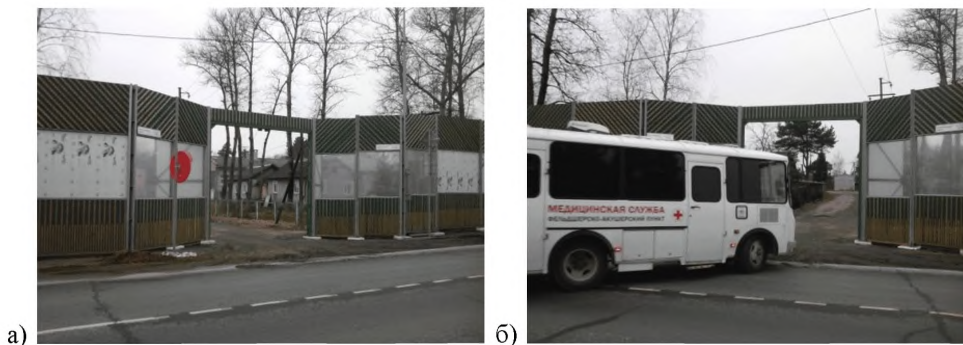
а – общий вид экрана с открытыми воротами, б – пример эксплуатации проезда Рисунок 13 – Пример организация разрыва в шумозащитном экране с устройством ворот и установкой дорожного зеркала на автомобильной дороге II категории с двумя полосами движения
