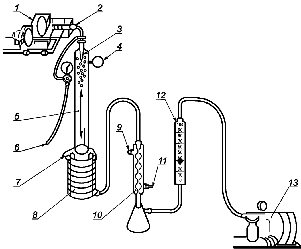
Рисунок В.1 — Принцип работы прибора для испытания эффективности бактериальной фильтрации
