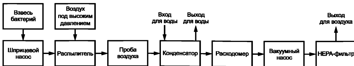
Рисунок В.1 — Принцип работы прибора для испытания эффективности бактериальной фильтрации
