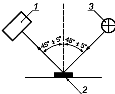
1 — блескомер или яркомер-блескомер; 2 — демаркированная разметка; 3 — источник света
