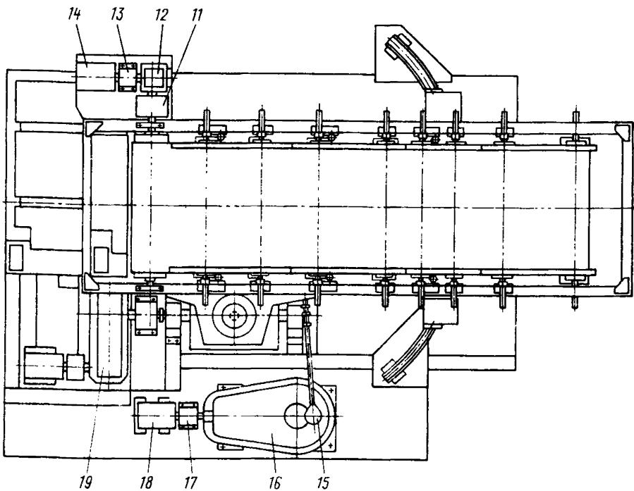
Рис. 14.1. Укладчик качающийся
