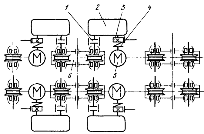
Рис. 19.2. Кинематическая схема механизма передвижения
