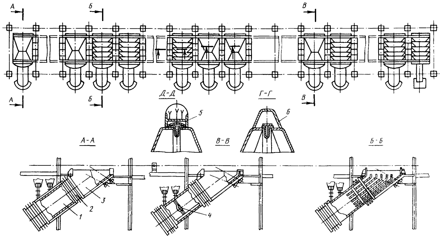
Рис. 16.9. Установка газоздушных камер
