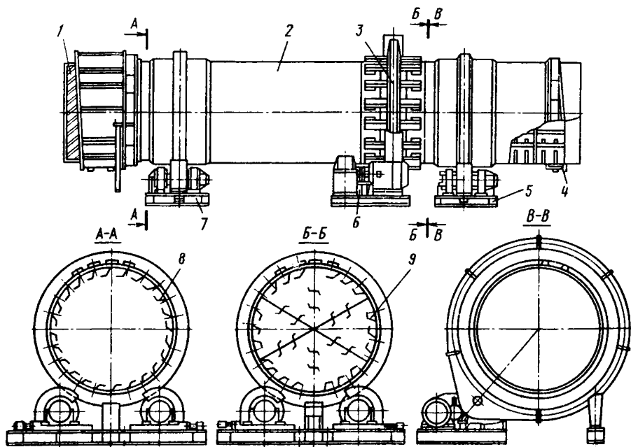
Рис. 6.1. Сушилка барабанная
