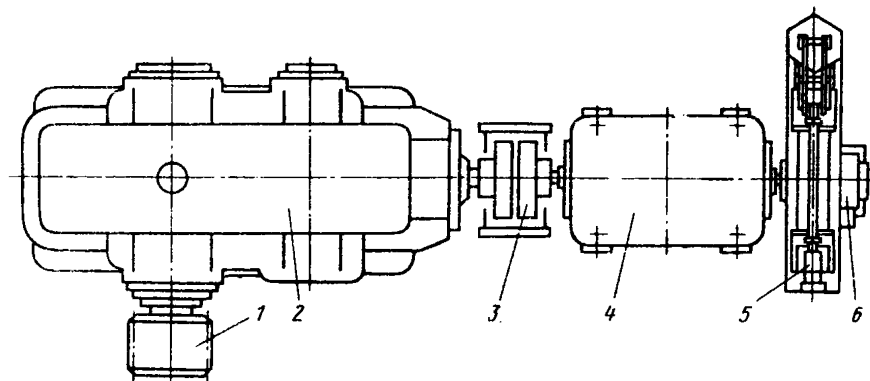
Рис. 11.2. Привод
