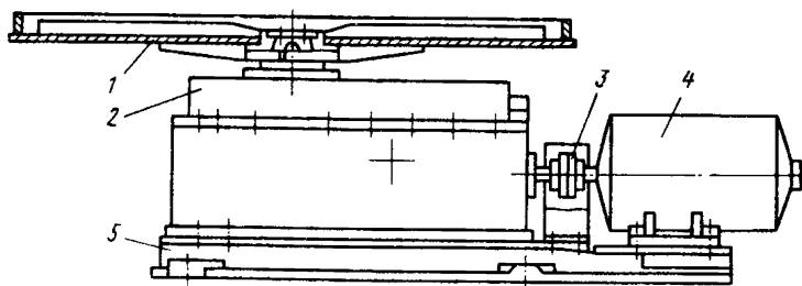
Рис. 9.1. Питатель дисковый
