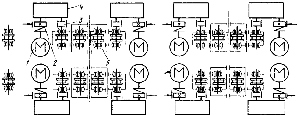
Рис. 18.6. Кинематическая схема механизма передвижения
