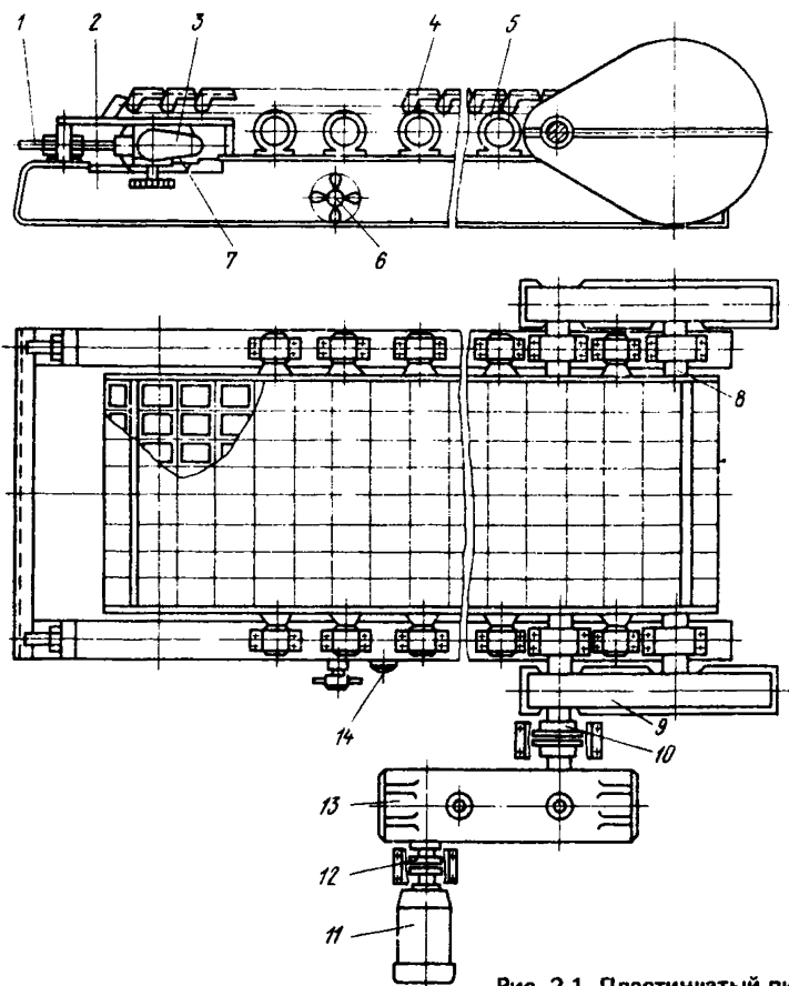
Рис. 2.1. Пластинчатый питатель
