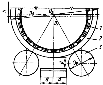
Рис. 6.6. Схема определения зазора между бандажом и прокладками:
