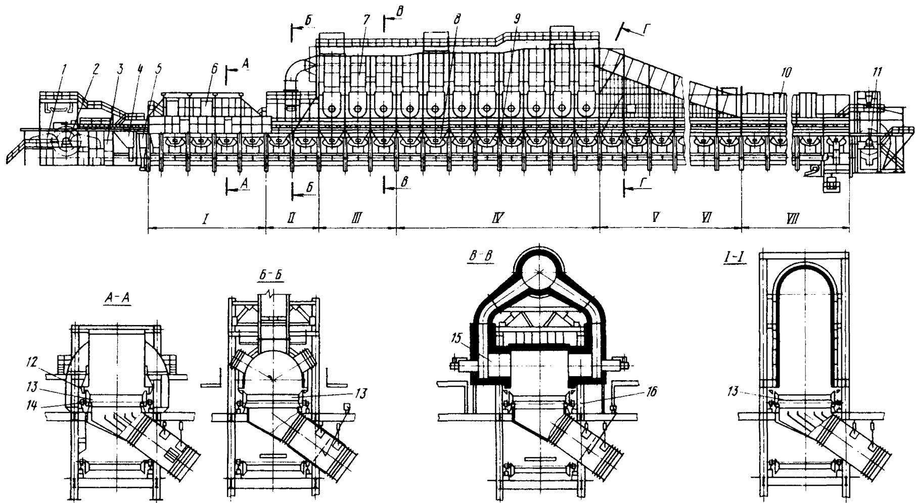
Рис. 16.1. Обжиговая машина:
