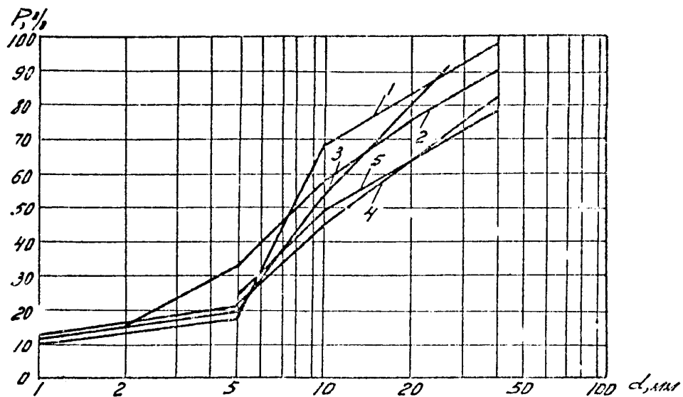
Рис.1. Типичные кривые зернового состава отходов углеобогащения с коксохимических заводов 1-Запорожский КХЗ; 2- Авдеевский КХЗ; 3-Днепродзержинский КХЗ; 4 -Ясиновский КХЗ; 5-Енакиевский КХЗ
