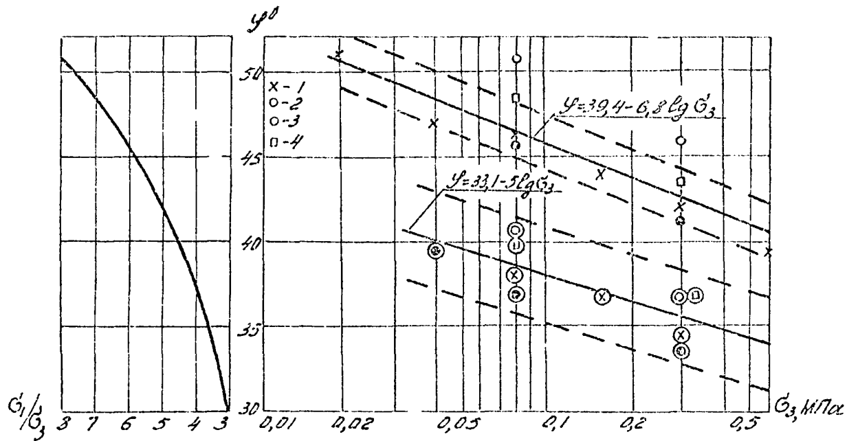
Рис.4. Зависимость угла внутреннего трения отходов углеобогащения коксохимических заводов от напряжений I-Днепродзержинский КХЗ; 2-Андреевский КХЗ, начальное состояние; 3- то же, конечное состояние; 4 - Енакиевский КХЗ
