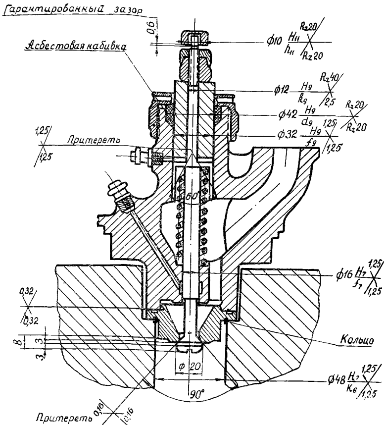
Рис. 4.6. Газовыпускной (инжекторный) клапан газомотокомпрессора 10ГК
