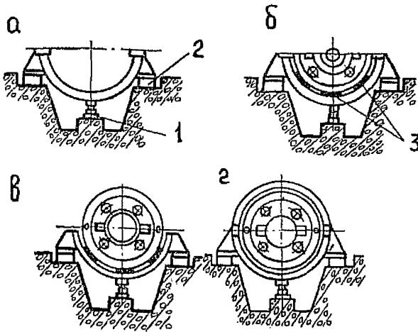
Рис. 3.40. Последовательность монтажа электродвигателя с разъемным статором. 1 — домкрат; 2 — фундаментная плита; 3 — картонные прокладки
