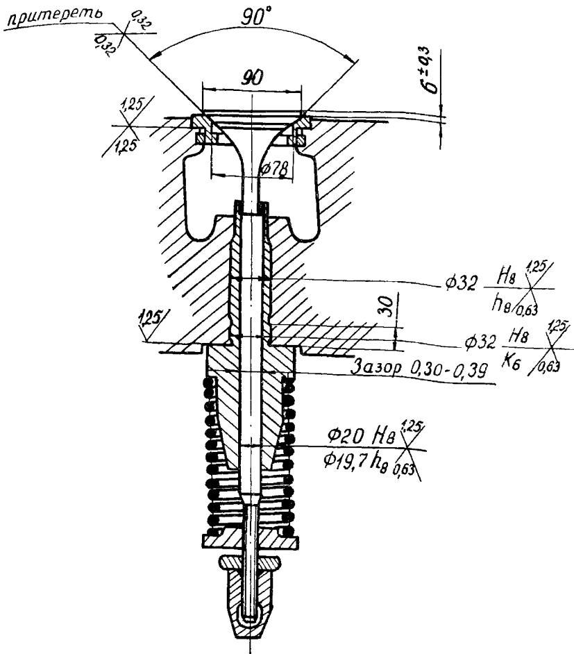
Рис. 4.5. Выпускной (впускной) клапан газомотокомпрессора 8ГК
