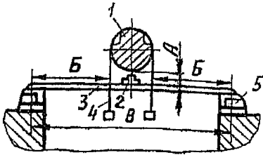
Рис. 3.39. Выверка плит статора на фундаменте. 1 — коленчатый вал; 2 — уровень; 3 — контрольная линейка; 4 — отвес; 5 — плита статора; А, Б — В — контрольные замеры
