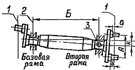
Рис. 3.8. Проверка перпендикулярности оси вала к оси ряда.
