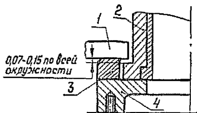
Рис. 3.35. Замер зазоров по торцу дроссельной втулки сальника. 1 — лишейка; 2 — дроссельная втулка; 3 — дистанционное кольцо; 4 — первая камера
