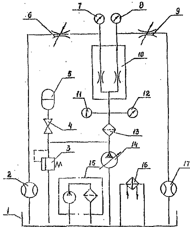
1 — гидробак; 2, 17 — расходомеры; 3 — предохранительный гидроклапан; 4 — вентиль; 5 — гидроаккумулятор; 6, 9 — гидродроссели; 7, 8, 12 — манометры; 10 — испытываемый гидроаппарат; 11 — термометр; 13 — фильтр; 14 — насос; 15 — фильтрующая установка; 16 — теплообменный аппарат
