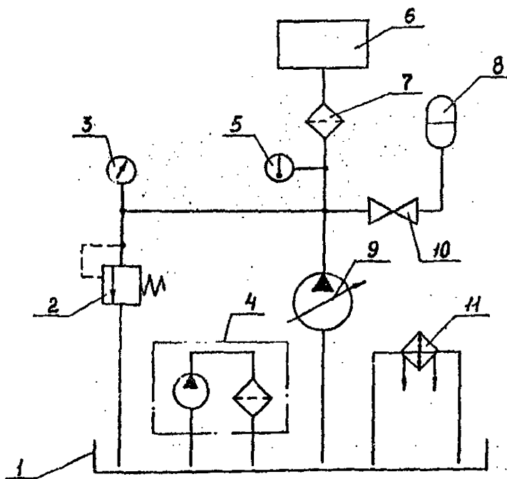
1 — гидробак; 2 — переливной гидроклапан; 3 — манометр; 4 — фильтрующая установка; 5 — термометр; 6 — испытываемый гидроаппарат; 7 — фильтр; 8 — гидракумулятор; 9 — насос; 10 — вентиль; 11 — теплообменный аппарат
