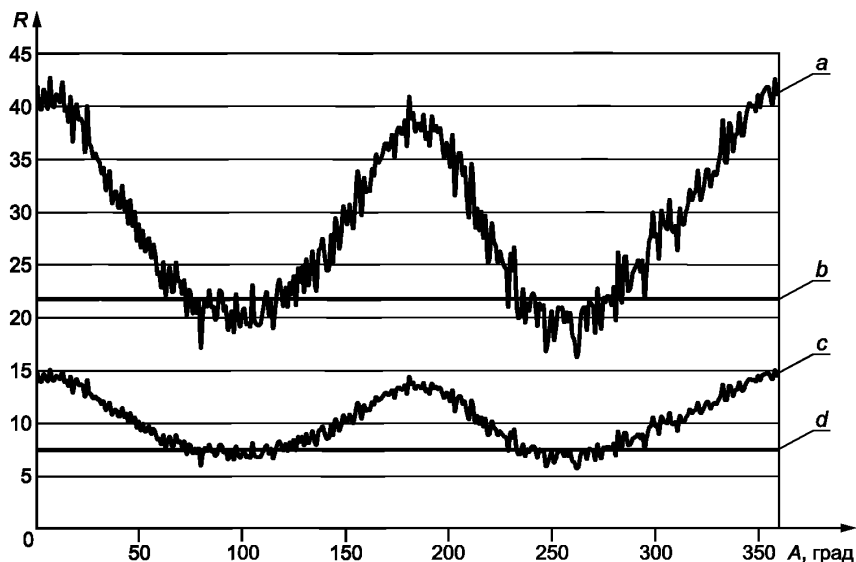
A — азимут, град; R — значение ЭПР, выраженное в квадратных метрах; a — 0° возвышение; b — SPL для 21,7 м 2 ; c — 10° возвышение; d — SPL для 7,5 м 2
