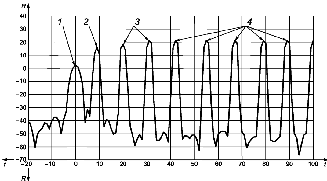
R — значение ЭПР, дБм 2 ; t — момент времени, нс; 1 — отражение от корпуса испытуемого оборудования; 2 — основной отраженный сигнал; 3 — ответные сигналы от испытуемого оборудования при увеличении возбуждения мощности сигнала; 4 — ответные сигналы от испытуемого оборудования в условиях насыщения
