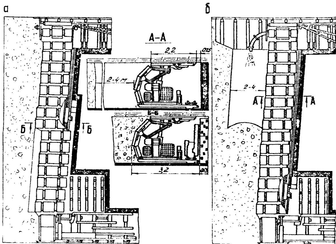
Рис. 6.5. Технологическая схема выемки угля и закладки выработанного пространства при применении комплекса КИК-1; а - начало цикла по выемке угля; б - закладка выработанного пространства
