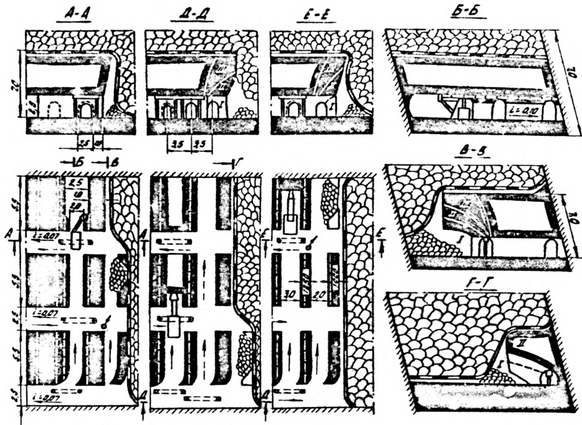
Рис. 4.6. Схема обработки угольного массива под глубоким перекрытием полосами по восстановлению с гидроотбойкой
