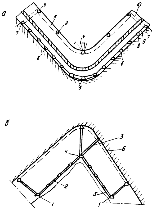
Рис. 3.9. Усовершенствованные схемы отработки синклинальных и антиклинальных замковых складок: а - схема отработки синклинальной складки по методу А.И.Широкова, В.Н.Замышляева, Л.С.Сенько, К.Ф.Санкина; б - то же, антиклинальной складки по методу А.П.Широкова, Л.И.Томашевского
