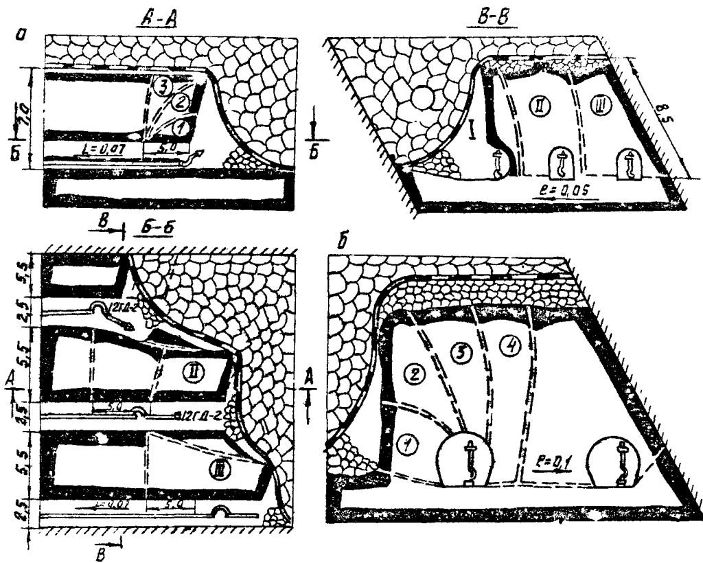
Рис. 4.4. Схема выемки угля в забоях с диагональным расположением гидромониторов: а - порядок выемки угля в подэтаже; б - последовательность выемки угля в заходке; I, II, III - номера подэтажей; 1, 2, 3, 4 - очередность выемки угля в заходке
