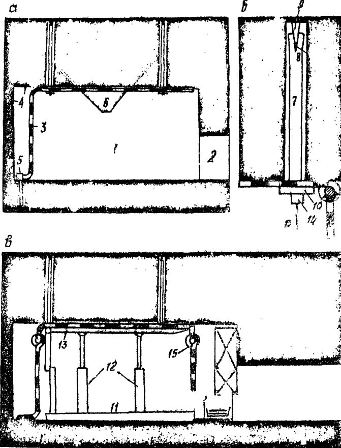
Рис. 6.7. Схема монтажа гибкого перекрытия: а - в монтажной раме; б - конструкция деревянного якера; в - в процессе выемки горизонтального слоя
