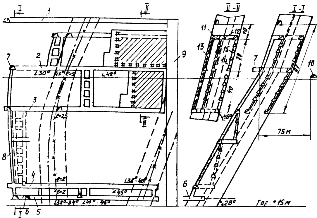
Рис. 3.12. Схема подготовки шлота Горелого на участке большой мощности; I - вентиляционный штрек; 2 - верхний промежуточный штрек; 3 - нижний промежуточный штрек; 4 - первый параллельный штрек; 5 - откаточный штрек; 6,7 - квершлаг; 8 - скат; 9 - профилактический цолик; 10 - полевой штрек; 11 - поперечно-наклонный слой; 12 - горизонтальный слой; 13 - монтажный слой; 14 - углеспускные печи; 15 - подэтажные штреки
