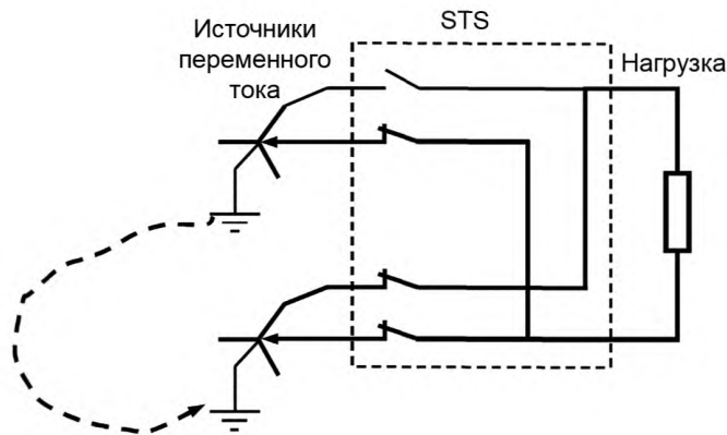
Рисунок D.2 — Перекрытие переключения нейтрали STS
