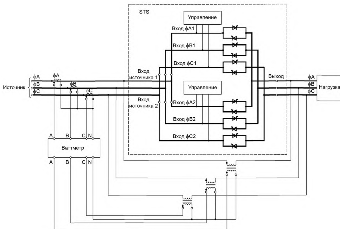
Рисунок 4 — Типовая схема для измерения потерь проводимости
