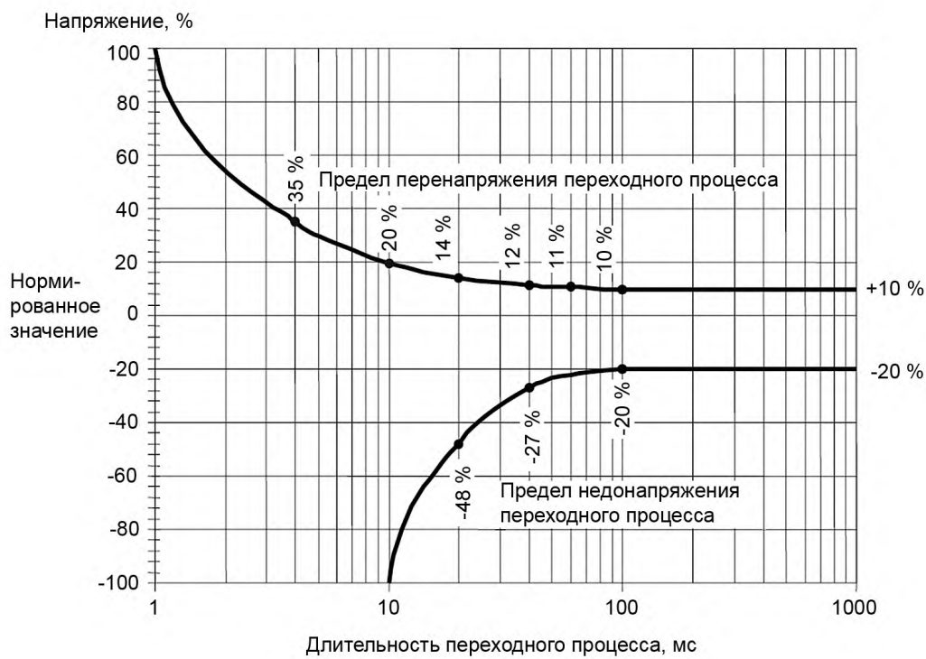
Рисунок В.3 — Допустимые отклонения источника классификации 3
