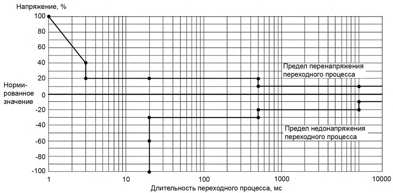
Рисунок В.4 — Допустимые отклонения источника классификации 4
