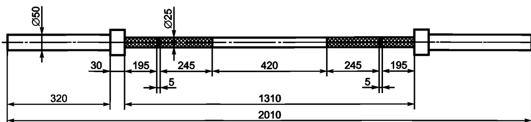
Рисунок 2 — Основные размеры женского грифа
