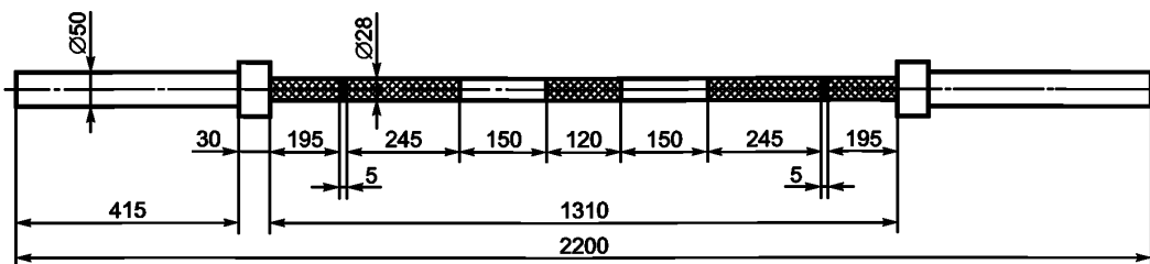
Рисунок 1 — Основные размеры мужского грифа
