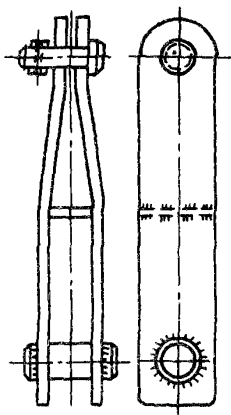
Серьги для подъема тяжелых грузов
