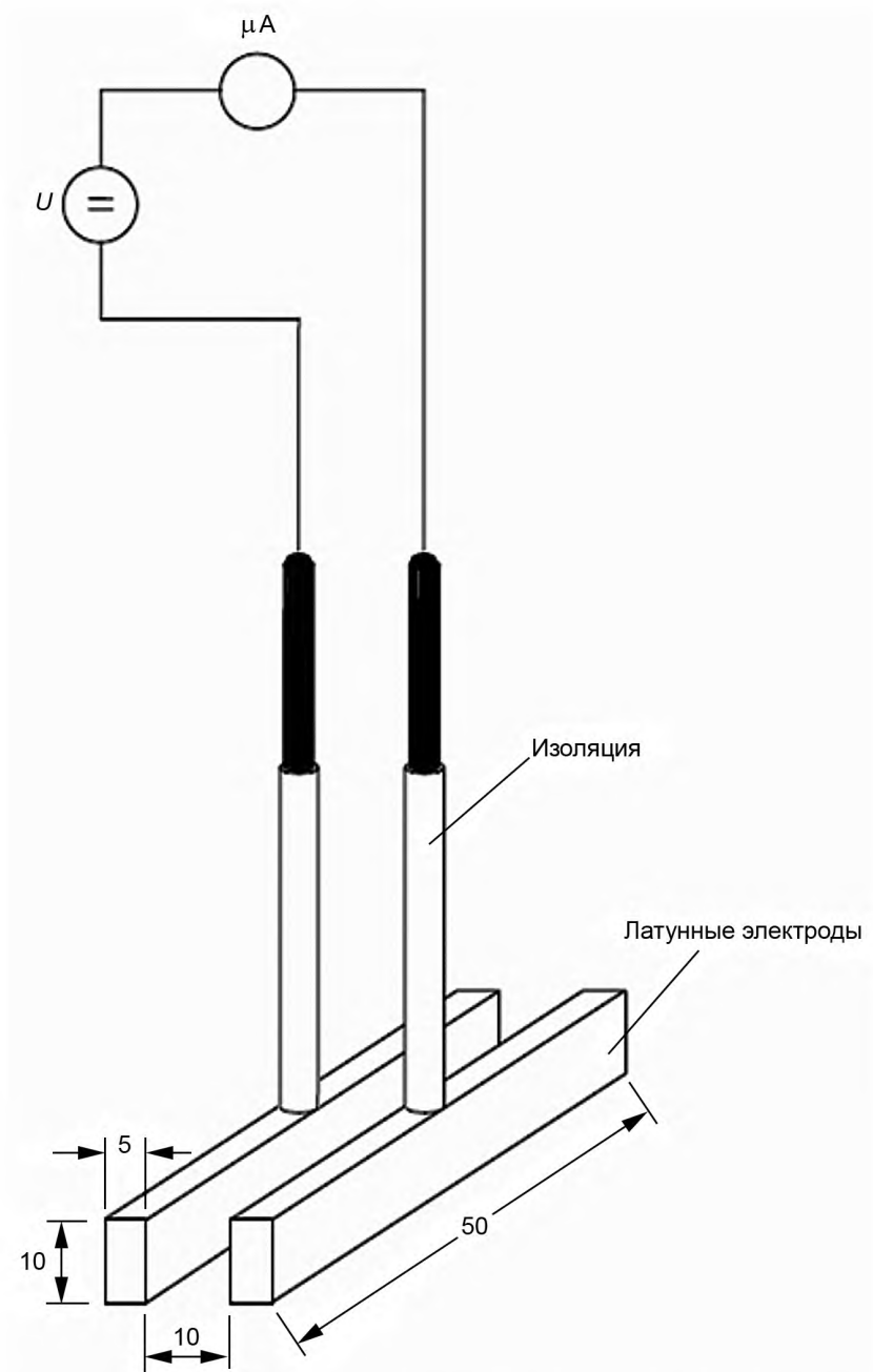
Рисунок 2 — Испытательная установка для определения электрической прочности заполнителя
