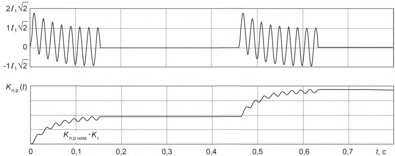
Рисунок Б.6 — Характер изменения потокоцепления в трансформаторе тока класса Р при отсутствии насыщения
