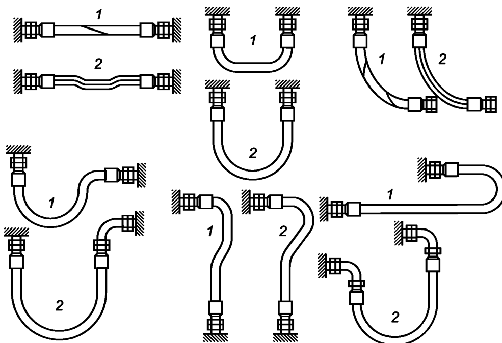
Рисунок 1 — Способы установки гибкого трубопровода: 1 — неправильно; 2 — правильно
