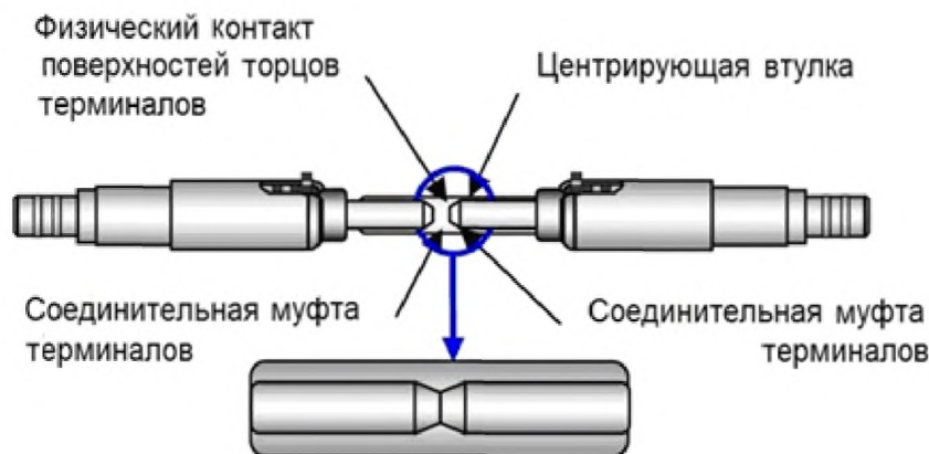
Рисунок 1 — Интерфейс и центровка волоконно-оптических терминалов
