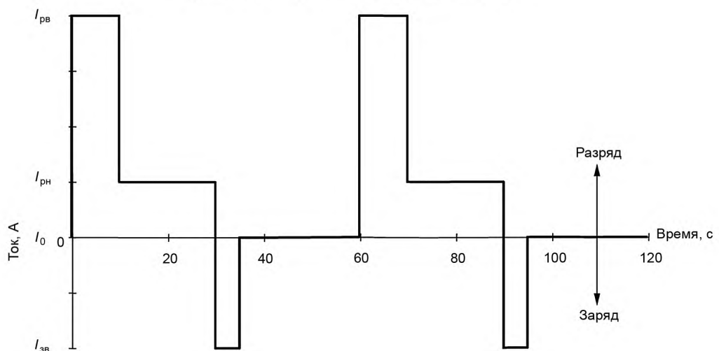
Рисунок 2 — Профиль испытания с рекуперацией
