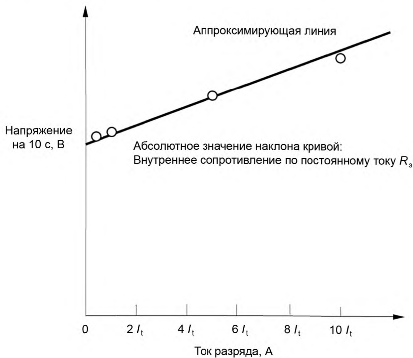
Рисунок А.7 — Метод получения значения внутреннего сопротивления по постоянному току при заряде
