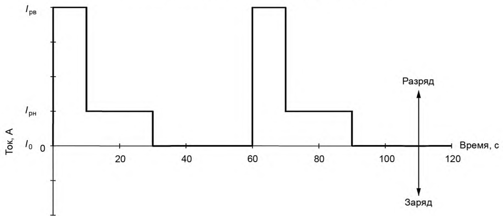
Рисунок 1 — Профиль испытания без рекуперации
